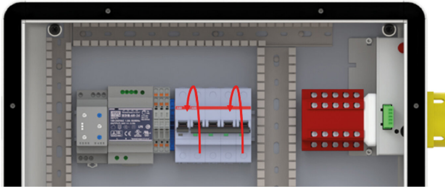
Abbildung 16. Einsichern der Leitungsschutzschalter in der AVU
