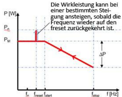
Abb. 178. Nicht-Hysterese
