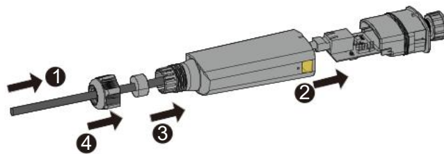
Abb. 46. LAN-Kabel durch Gehäuse führen und LAN-Stecker anschließen und Dichtung anbringen
