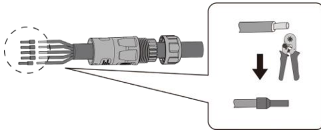
Abb. 16. Crimpen Sie die Aderendhülse an den Kontakt.
