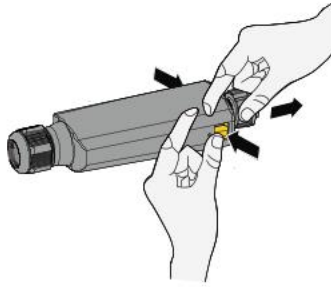
Abb. 45. Entriegelungsflaschen an Kommunikationseinheit eindrücken
