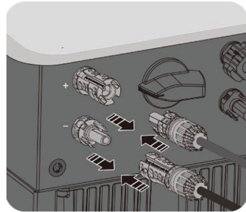
Abb. 41. Verbinden der Batterie-Anschlüsse
