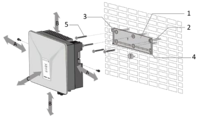
Abb. 9. Montage der Wandhalterung
