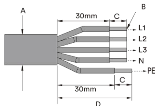
Abb. 15. Isolieren Sie die Drähte ab.
