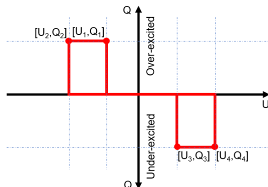
Abb. 199. Q(U)-Kurve und Hysterese
