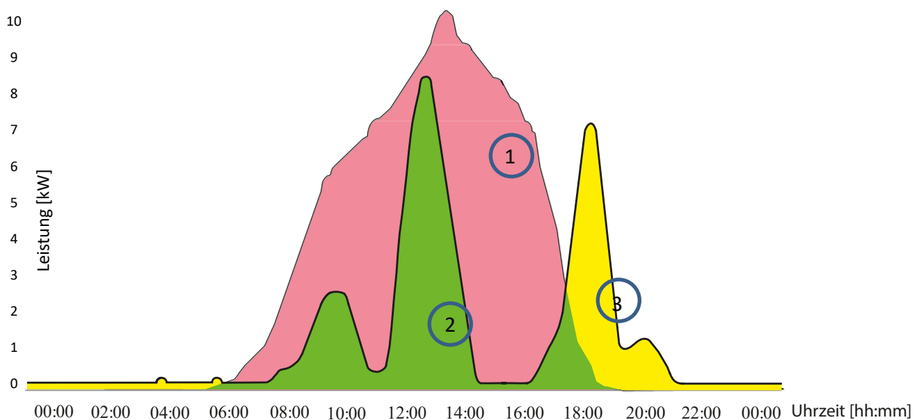
Abb. 241. Diagramm zur 0% Regelung
