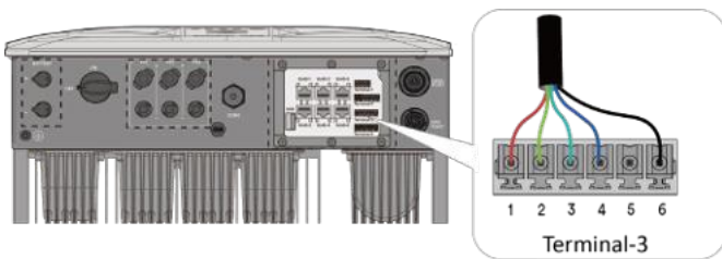
Abb. 60. Netzwerkkabel anschließen
