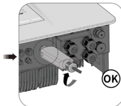
Abb. 44. Anschluss der Kommunikationseinheit
