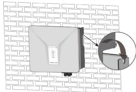
Abb. 11. Sicherer Sitz des Geräts prüfen
