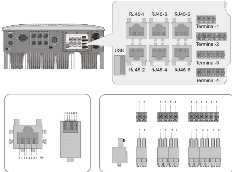
Abb. 49. Anschluss und Belegung der Schnittstellen
