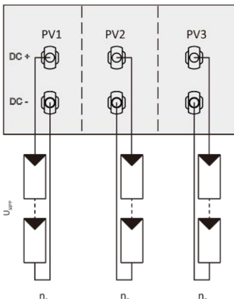
Abb. 32. Zuweisung aller MPP-Tracker
