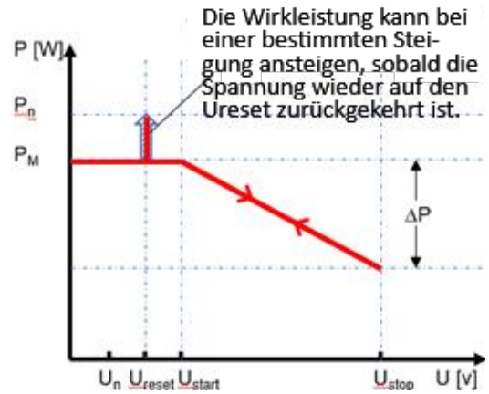
Abb. 183. Nicht-Hysterese
