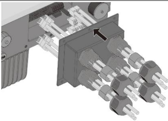
Abb. 53. Befestigen Sie das Kommunikationskabel an den entsprechenden Terminals
