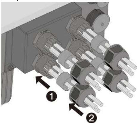
Abb. 55. Mutter anziehen
