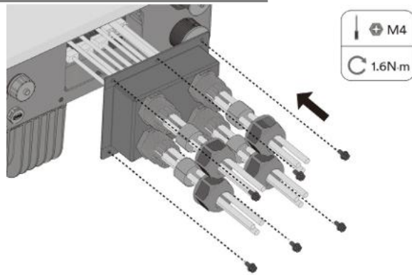
Abb. 54. Befestigen Sie die AC/COM-Abdeckung
