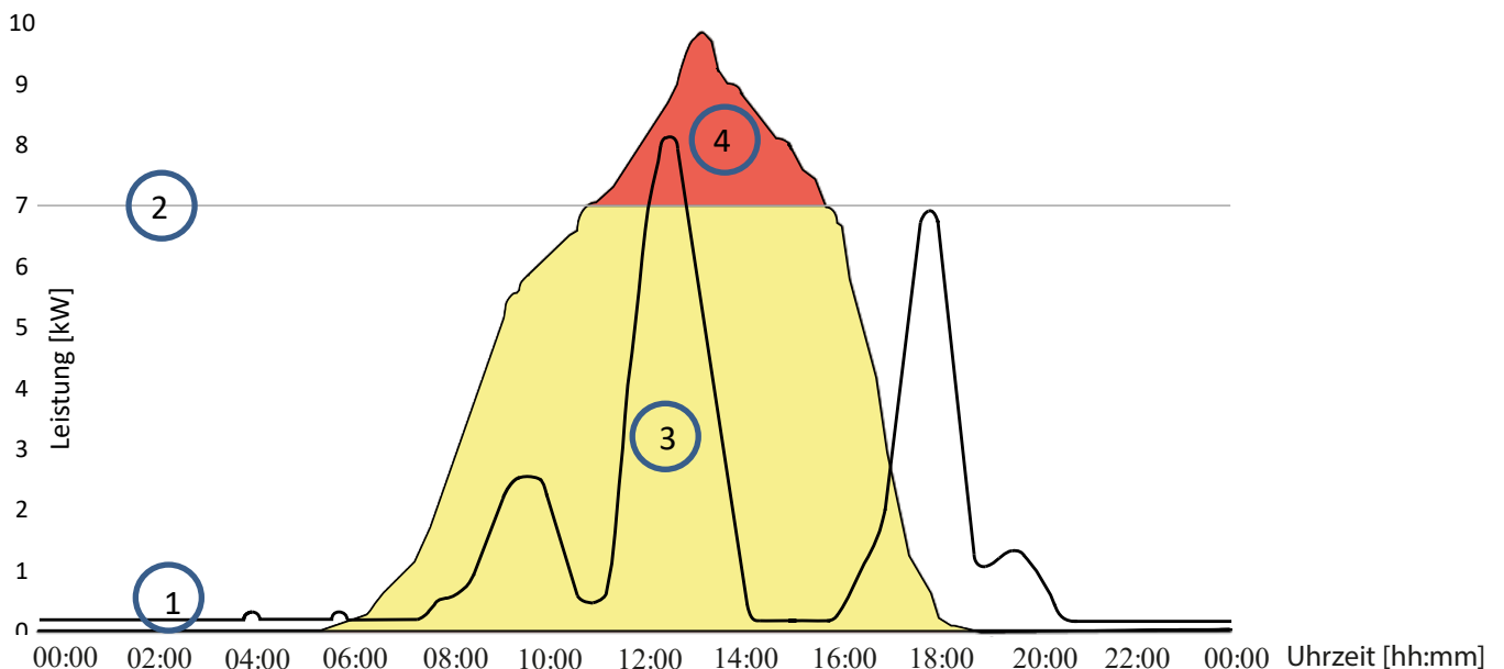
Abb. 239. Diagramm zum Vergleich zwischen Energiebedarf Einfamilienhaus und PV-Leistung
