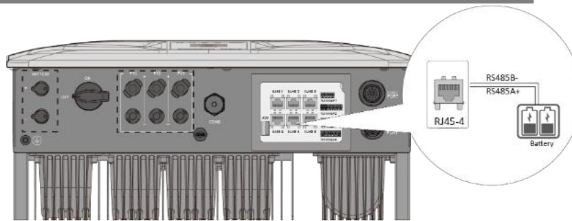
Abb. 57. Anschluss BMS Kommunikation
