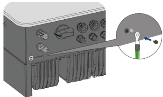
Abb. 42. Erdung anschließen
