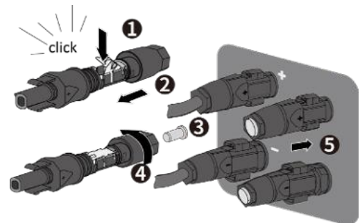
Abb. 35. Setzen Sie die DC-Steckverbinder ein und verschließen Sie ungenutzte Steckverbinder
