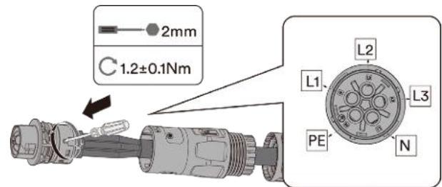
Abb. 24. Kabel am Kontaktträger befestigen
