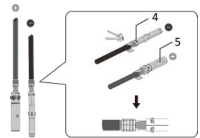
Abb. 38. Kabelenden mit der Crimpzange vorbereiten.
