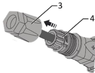
Abb. 30. Einsatz in Hülse schieben
