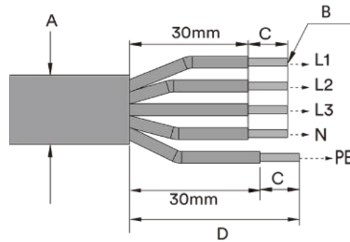
Abb. 22. Isolieren Sie die Drähte ab.
