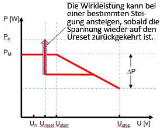
Abb. 184. Hysterese
