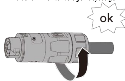
Abb. 24. Kabel am Kontaktträger befestigen
