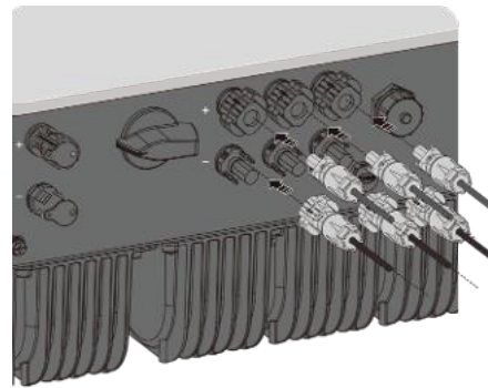
Abb. 34. Strombelastbarkeit und PV-Anschluss
