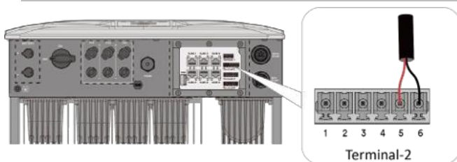
Abb. 58. Netzkabel anschließen
