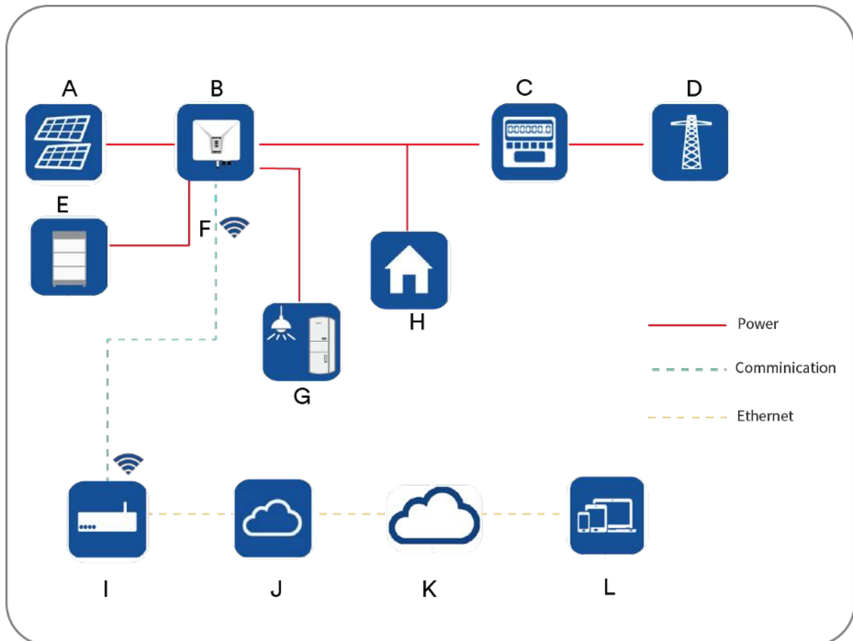
Abb. 2. Systemdiagramm.
