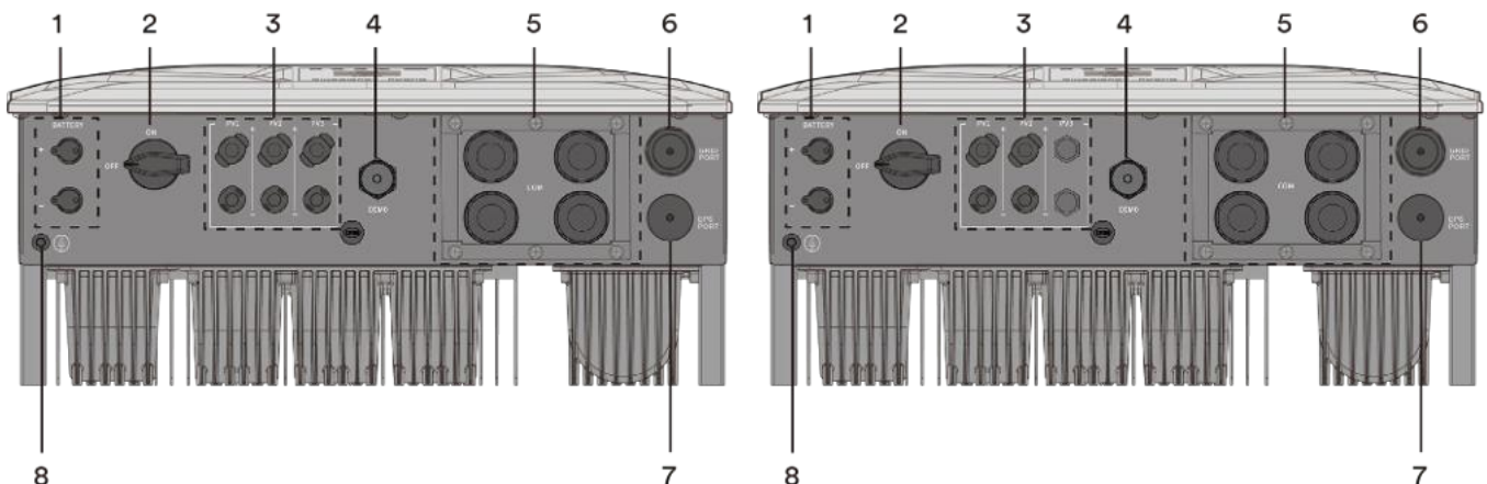
Abb. 13. mit 3 MPPT (links) / mit 2 MPPT (rechts)
