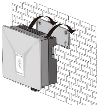
Abb. 10. Wechselrichter in die Wandhalterung einsetzen
