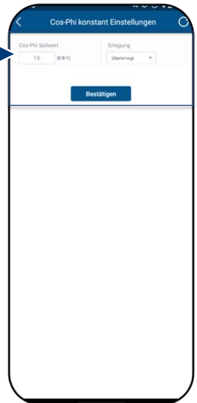
Abb. 190. Bestimmen des <Cos-phi> Zielwerts
