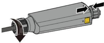
Abb. 47. Kabelverschraubung befestigen
