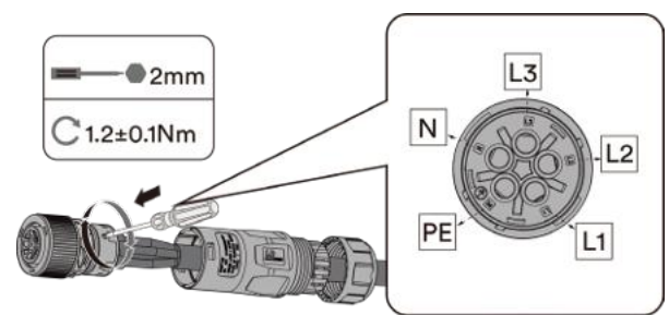
Abb. 17. L1-L3 & N+PE einführen und festziehen
