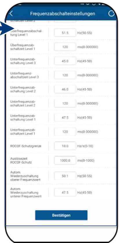
Abb. 143. Frequenzbereich und ROCOF-Schutzgrenze einstellen
