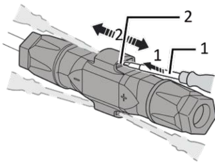
Abb. 248. Steckverbinder abstecken
