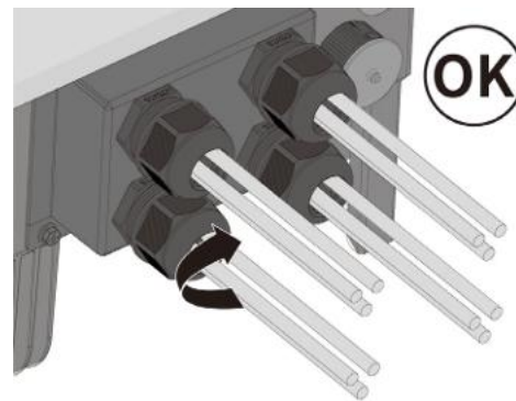
Abb. 54. Befestigen Sie die AC/COM-Abdeckung
