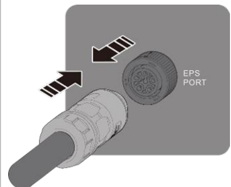
Abb. 27. Verbinden der Anschlüsse
