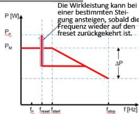
Abb. 179. Hysterese
