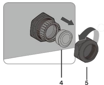
Abb. 51. Kabelverschraubungen für Kommunikationskabel
