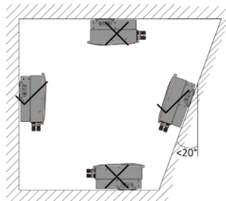
Abb. 5. Erlaubte Aufstelllage
