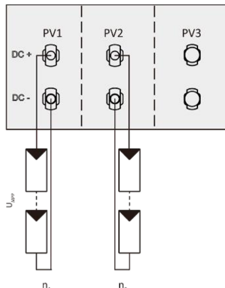
Abb. 33. Zuweisung von nur zwei MPP-Trackern
