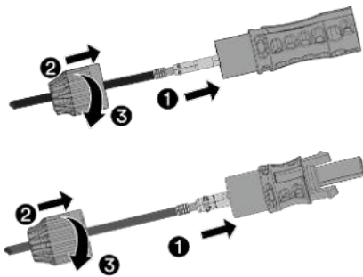
Abb. 39. Anziehen der Kabel
