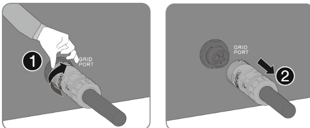
Abb. 244. Lösen und entfernen Sie den AC-Anschluss.
