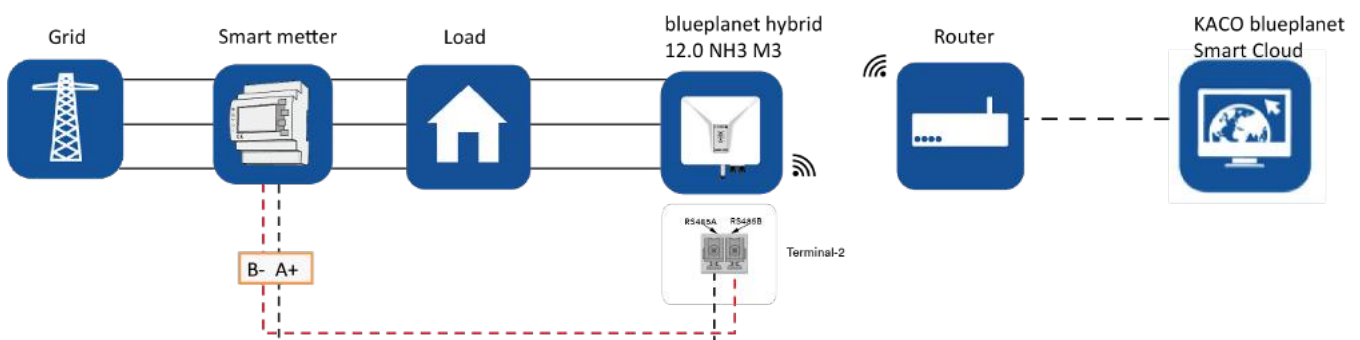
Abb. 111. Blockdiagramm für dynamische Einspeisung bei Auswahl von SDM630CT
