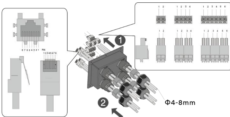
Abb. 52. Kommunikationsleitungen über Kabel
