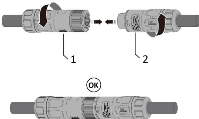
Abb. 28. Bypass Anschluss
