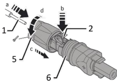
Abb. 29. Adern einfügen
