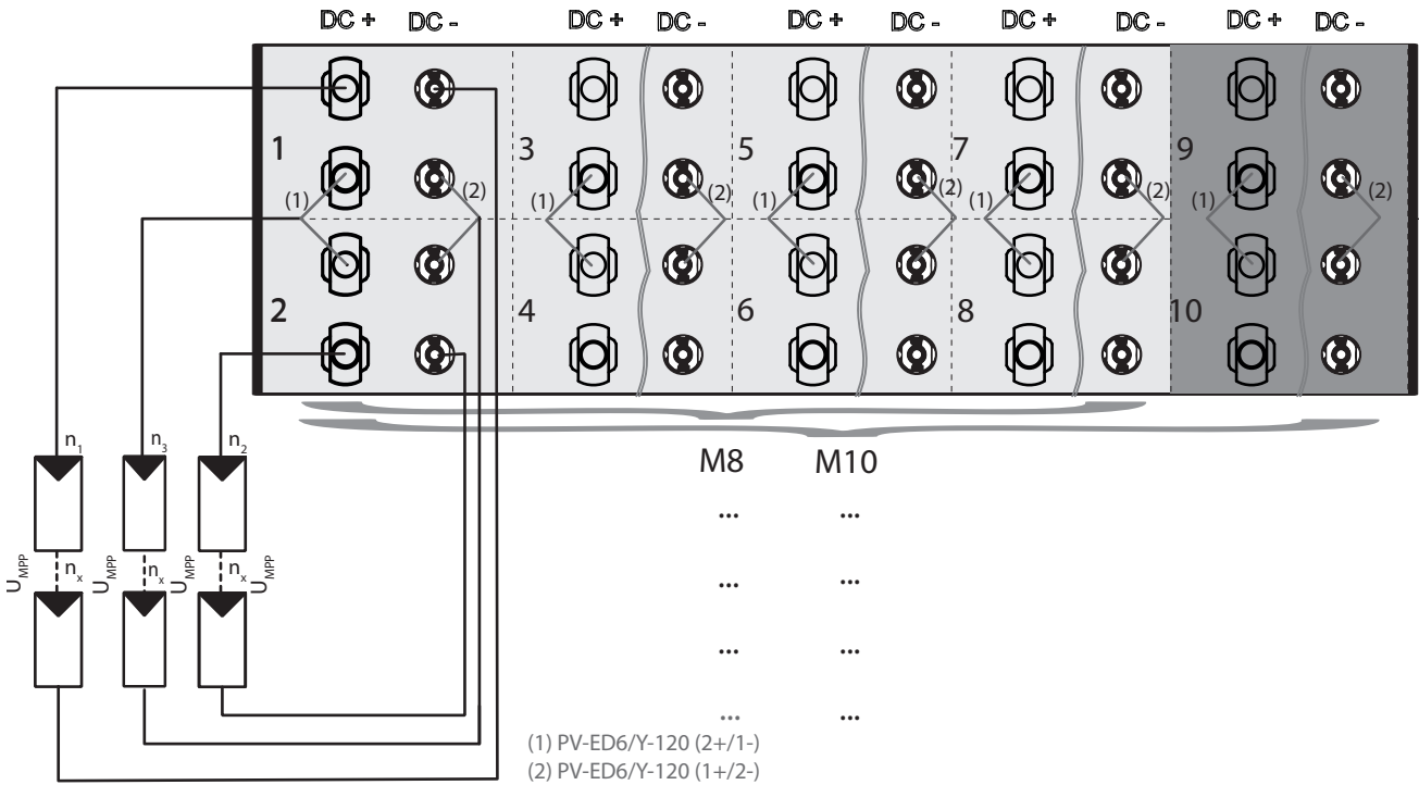
Abb. 35: Anschlussschema: 1 String parallel über 2 MPP-Tracker und je 1 String getrennt auf je 1 MPP-Tracker
