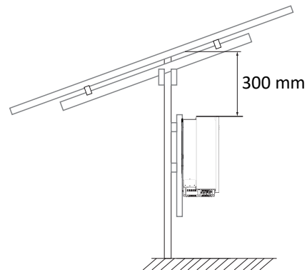
Abb. 15: Anbauhinweis unter PV-Anlage
