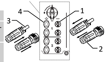
Abb. 39: Anschluss an Steckverbinder
