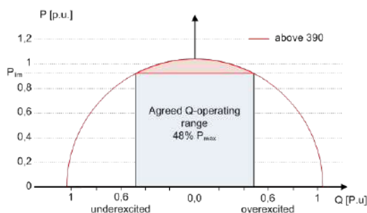
Abb. 83: P-Q-Betriebsbereich mit begrenzter Wirkleistung ( Q_{max}=S_{max} \neq P_{max} ) für PV-Wechselrichter
