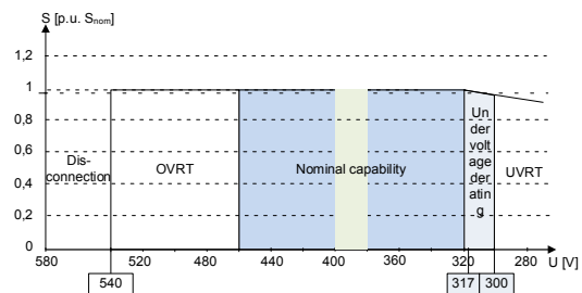
Abb. 68: Scheinleistung abhängig der Netzspannung für blueplanet 100 NX3
