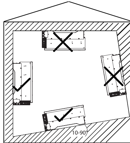
Abb. 13: Erlaubte Aufstelllage
