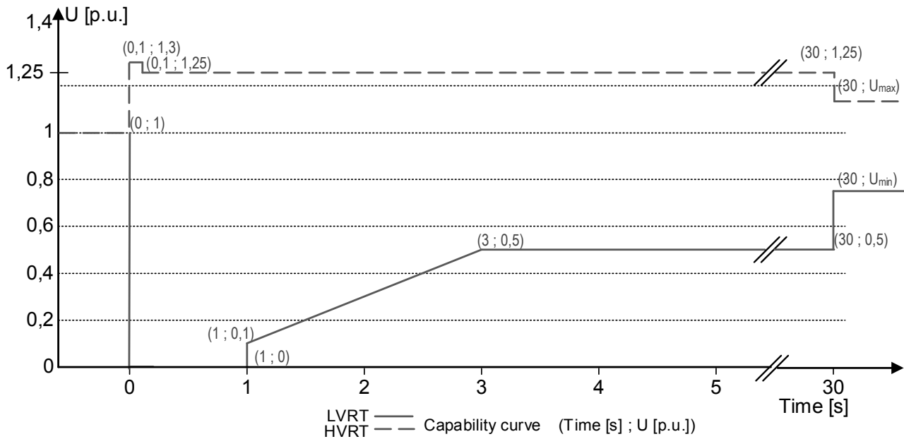
Abb. 82: Störfestigkeitskennlinie bezogen auf die Nennspannung
