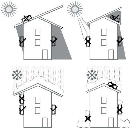
Abb. 12: Gerät bei Außeninstallation
