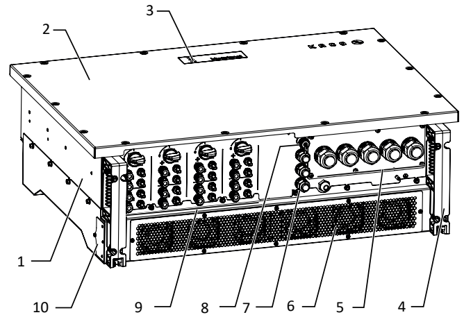
Abb. 4: Aufbau des Gerätes (M8-Variante)
