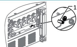
Abb. 40: Zusätzlicher Erdungspunkt
