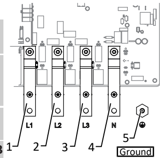
Abb. 29: AC-Netzanschluss 4/5-polig
