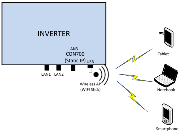
Abb. 49: Inbetriebnahme über WiFi Direktverbindung
