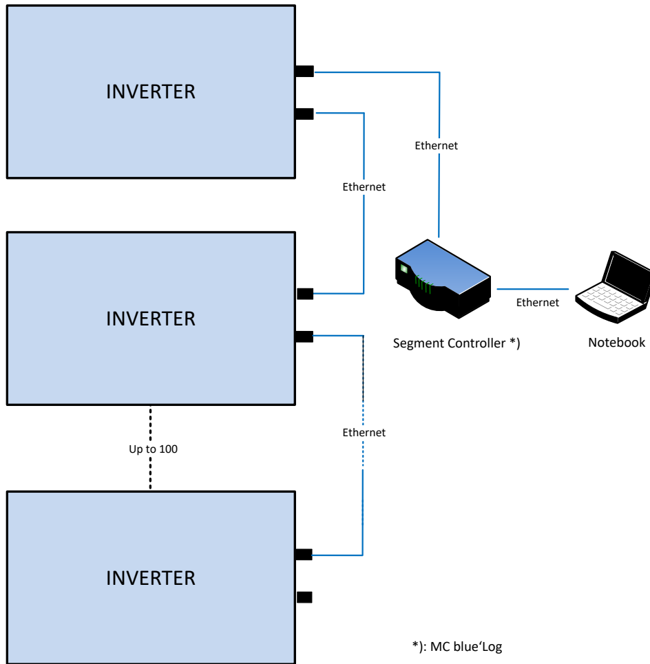
Abb. 53: Inbetriebnahme über Segment Controller
