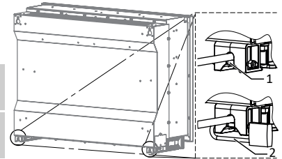
Abb. 96: Gerät mit Vorhängeschloss absichern
