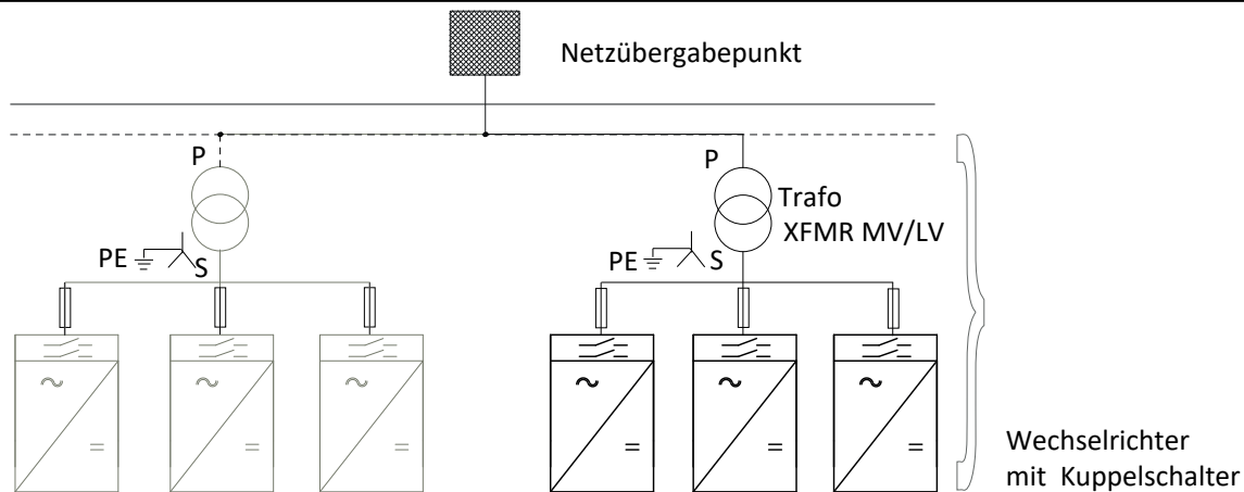
Abb. 7: Übersichtsschaltplan vom Netzübergabepunkt zum Wechselrichter
