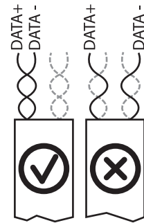
Abb. 44: Belegung der verdrehten Adernpaare
