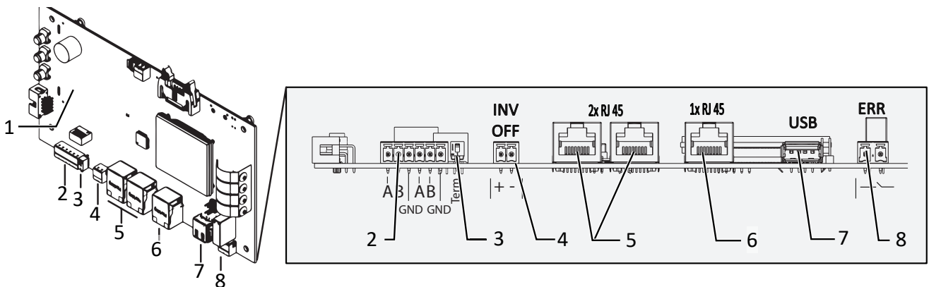
Abb. 41: Kommunikationsplatine (HMI-Platine)
