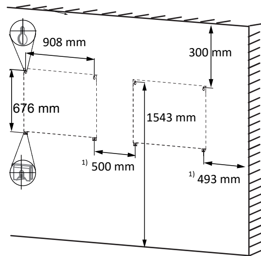
Abb. 20: Mindestabstände für Wandmontage
