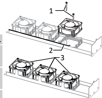
Abb. 89: Lüfter ausbauen
