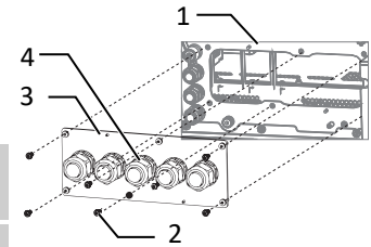
Abb. 27: AC-Eingangsplatte lösen
