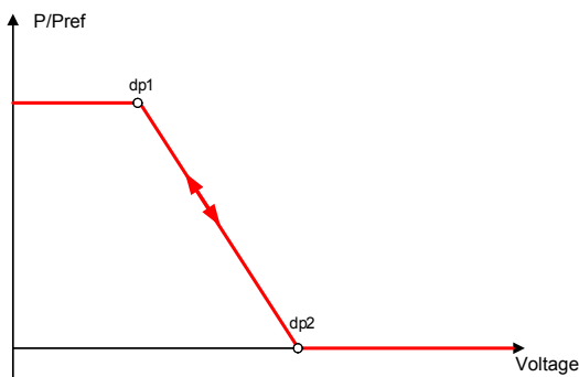
Abb. 74: Beispiel-Kennlinie ohne Hysterese
