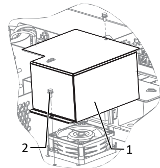
Abb. 90: Abdeckung vom ersten Innenraumlüfter lösen
