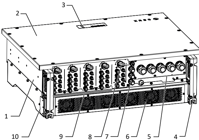
Abb. 3: Aufbau des Gerätes (M10-Variante)
