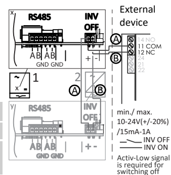
Abb. 45: Gerät mit externem Netzschutzgerät verbinden
