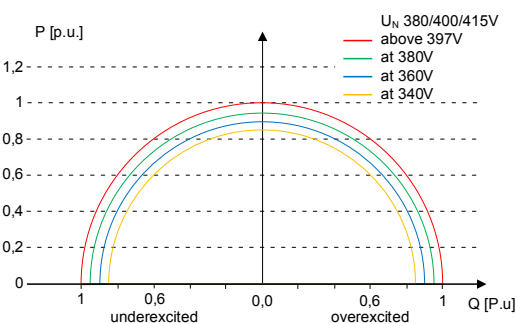
Abb. 69: P-Q Betriebsbereich für bp 125 NX3 ( Q_{max}=S_{max} )
