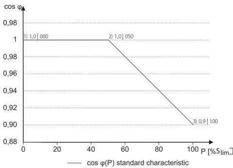
Abb. 71: \cos \varphi(P) Standard Kennlinie mit 3 Stützstellen
