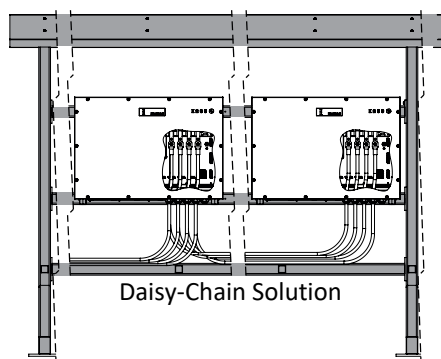
Abb. 14: Freiflächenmontage unter PV-Anlage
