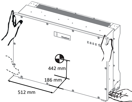
Abb. 21: Gehäuse anheben
