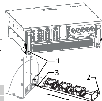
Abb. 87: Lüfterschublade öffnen
