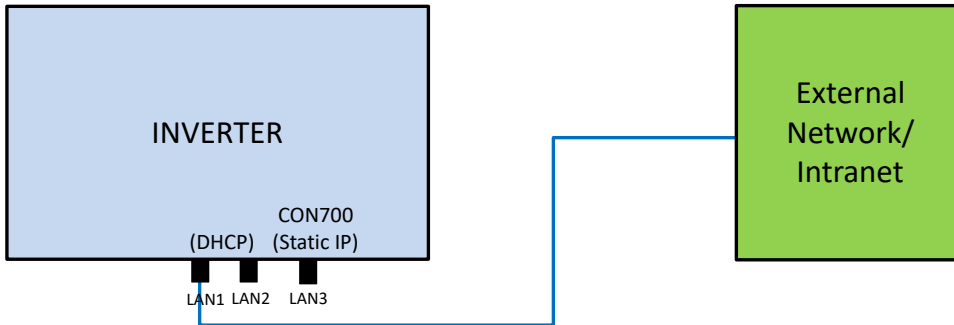
Abb. 52: Inbetriebnahme über externes Netzwerk ohne Segment Controller
