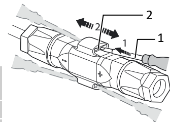
Abb. 95: Steckverbinder abstecken
