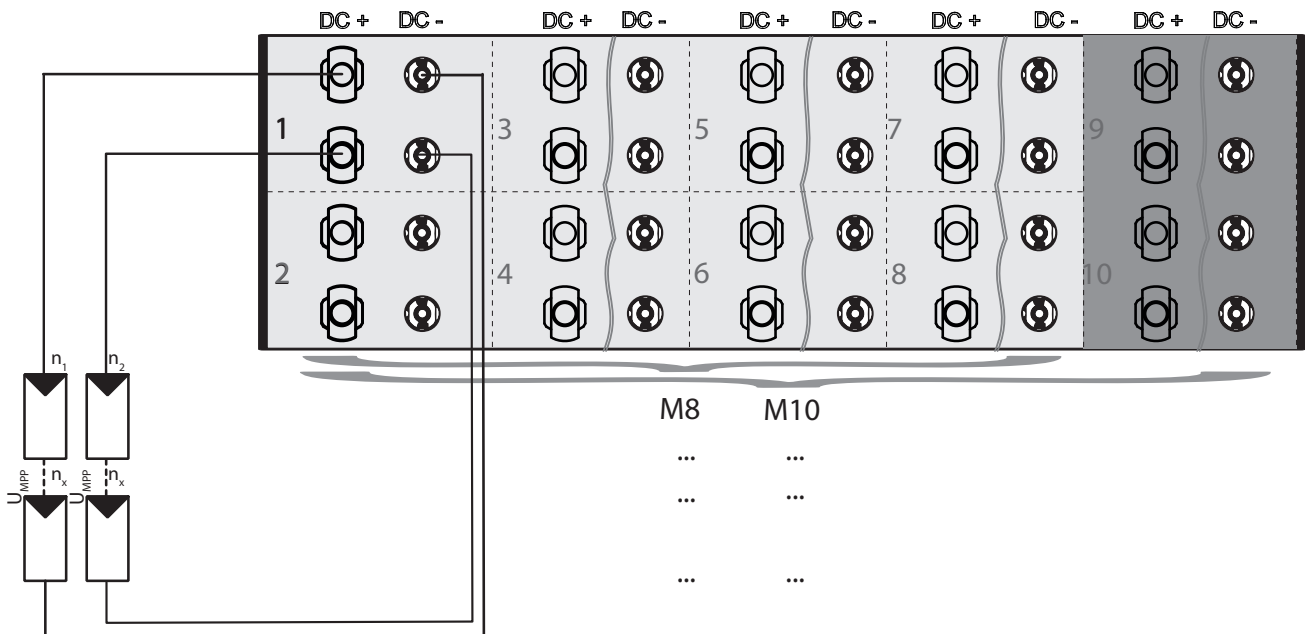
Abb. 30: Anschlussvariante: Jeweils 2 Strings an einen MPP-Tracker
