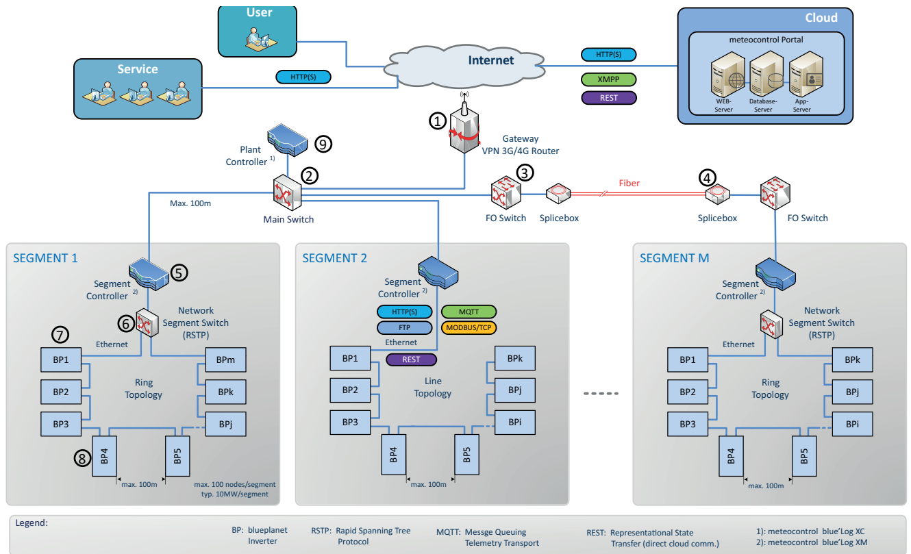
Abb. 48: Segmentierung einer Anlage
