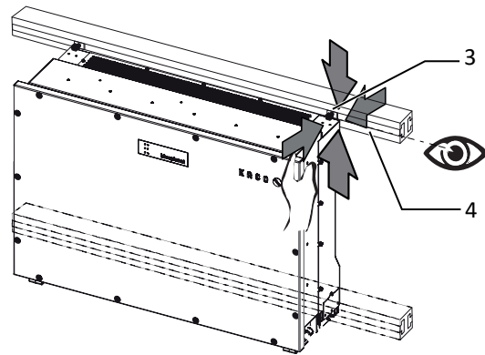
Abb. 22: Gerät in PV-Shelterprofil einhängen
