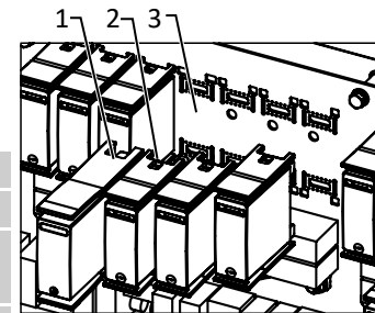
Abb. 94: DC Überspannungsschutz wechseln
