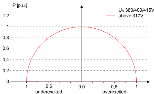
Abb. 67: P-Q Betriebsbereich für bp 100 NX3 ( Q_{max}=S_{max} )
