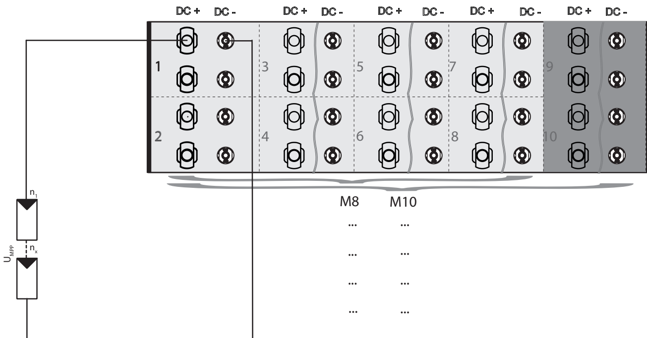
Abb. 32: Anschlussvariante: Jeweils 1 String an einen MPP-Tracker
