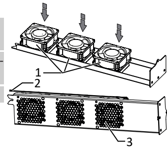
Abb. 88: Lüfterschublade reinigen
