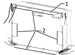
Abb. 24: Gehäusedeckel abnehmen
