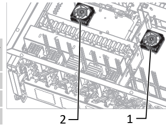
Abb. 92: Innenraumlüfter lösen
