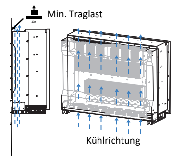
Abb. 11: Tragfähigkeit & Kühlrichtung
