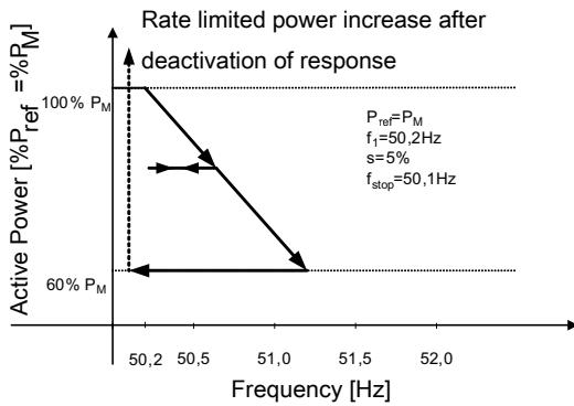
Abb. 80: Beispielverhalten mit Hysterese (Modus 1)
