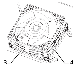
Abb. 91: Innenraumlüfter ausbauen
