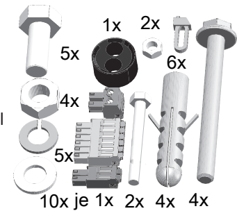
Abb. 8: Montagesatz
