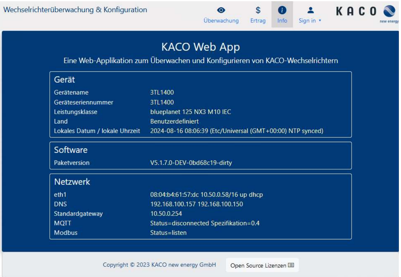
Abb. 66: Oberfläche für Geräte- und Hardwareinfos
