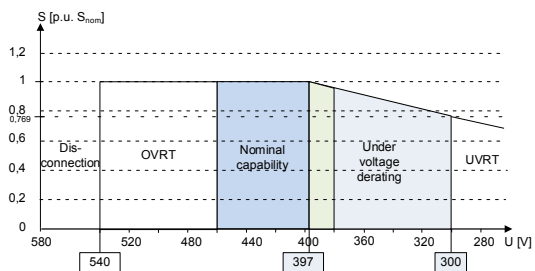
Abb. 70: Scheinleistung abhängig der Netzspannung für blueplanet 125 NX3
