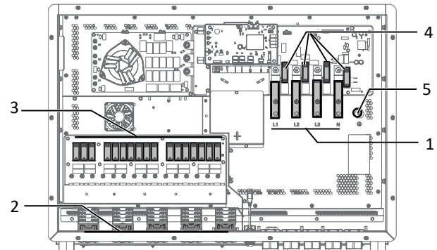
Abb. 26: Anschlussbereich M10-Version
