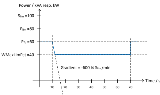
Abb. 84: Leistungsgradient gemäß Musterparameter und Berechnung
