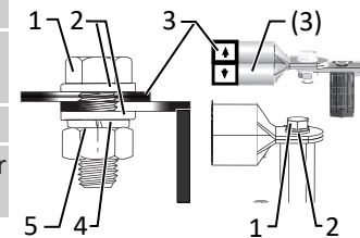
Abb. 28: AC-Anschluss vorbereiten
