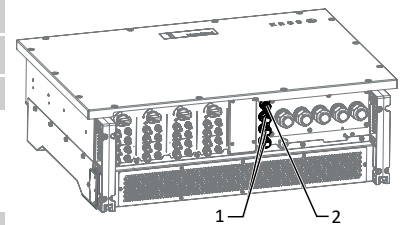
Abb. 42: Schnittstellenleitung einführen
