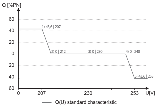
Abb. 72: Q(U) Standard Kennlinie mit 5 Stützstellen
