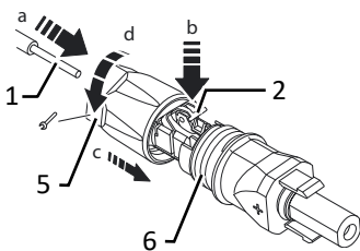
Abb. 36: Adern einfügen
