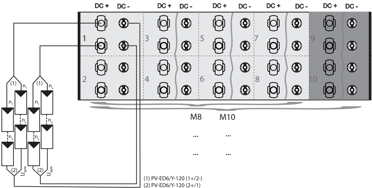
Abb. 34: Anschlussvariante: Jeweils 2 Strings über Y-Kabel an einen MPP-Tracker
