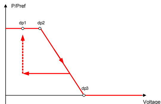
Abb. 75: Beispiel-Kennlinie mit Hysterese und einer Deaktivierungsschwelle unterhalb der Aktivierungsschwelle
