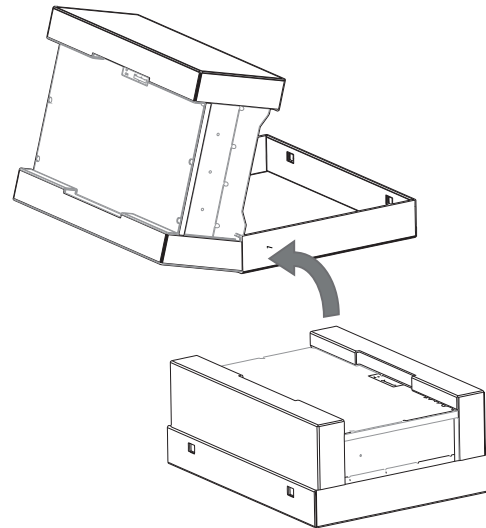
Abb. 17: Gerät aufrichten
