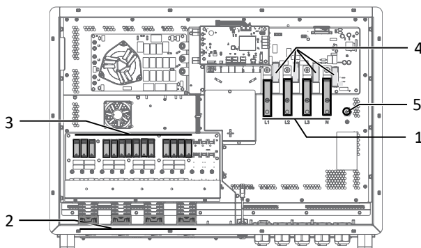
Abb. 25: Anschlussbereich M8-Version
