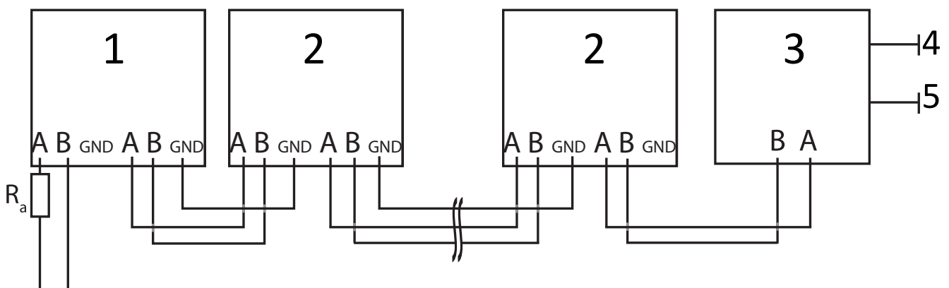
Abb. 43: Anschlussschema der RS485-Schnittstelle
