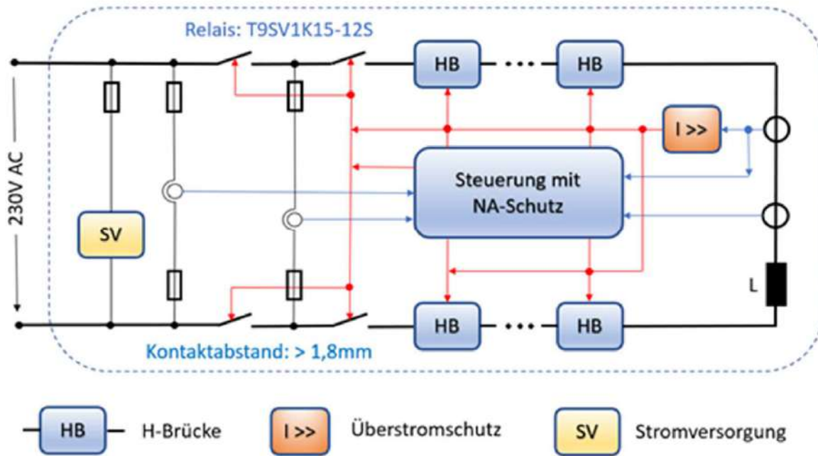
Abb. 12 Innenschaltung des Speichers
