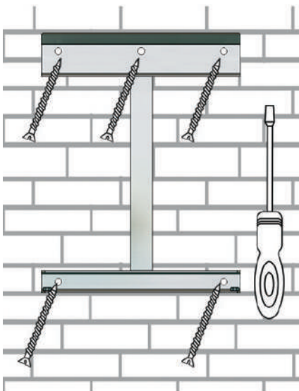
Abb. 16 Wandhalterung fixieren
