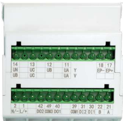
Abb. 41 ADW200: Draufsicht
