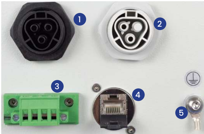
Abb. 9 Speicher von Unten (Steckplätze)
