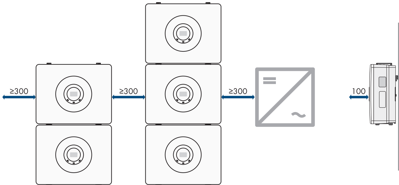
Abbildung 9: Empfohlene Abstände (Maßangaben in mm)
