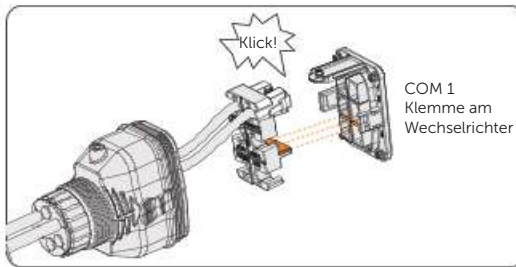
Abbildung 7-34 Den Steckverbinder an COM 1 einsetzen
