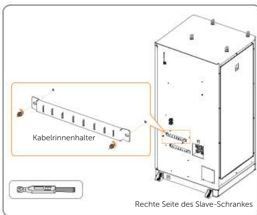
Abbildung 14-72 Kabelbinderhalterung entfernen
