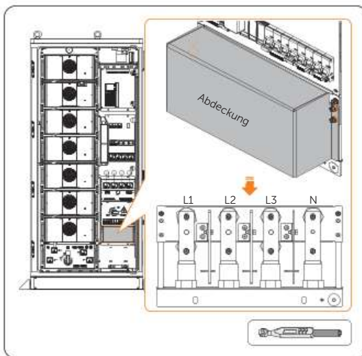
Abbildung 14-54 Abdeckung entfernen
