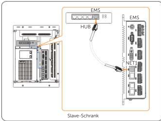
Abbildung 14-65 Kabel ausziehen
