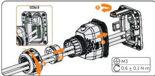
Abbildung 7-56 An den Wechselrichter anschließen
