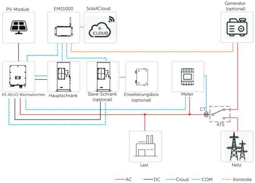
Abbildung 2-1 Systemübersichtdiagramm
