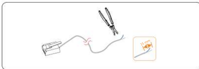
Abbildung 14-17 Kommunikationkabel für Meter abisolieren
