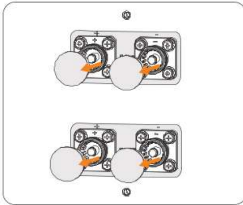
Abbildung 7-25 Batterieabdeckungen entfernen
