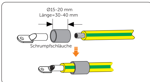
Abbildung 7-3 Schrumpfschläuche schneiden
