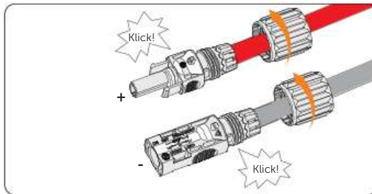
Abbildung 7-18 PV-Kabel sichern
