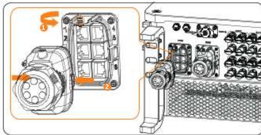
Abbildung 7-28 Das Steckverbindergehäuse entfernen
