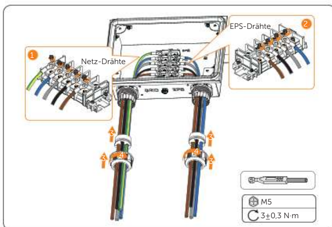
Abbildung 14-80 NETZ- und EPS-Drähte anschließen
