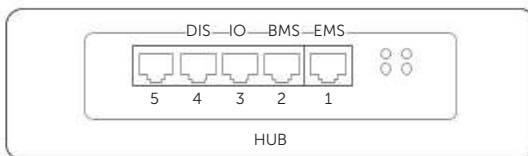
Abbildung 14-96 Beschreibung von HUB
