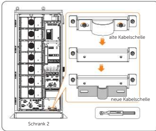
Abbildung 14-52 Klammer öffnen
