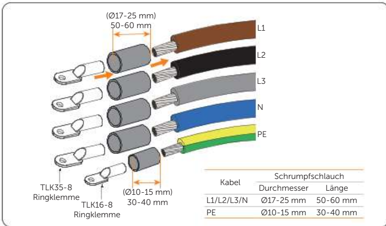
Abbildung 7-71 Schrumpfschläuche schneiden
