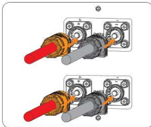
Abbildung 7-26 Montierte Batterieabdeckungen anschließen
