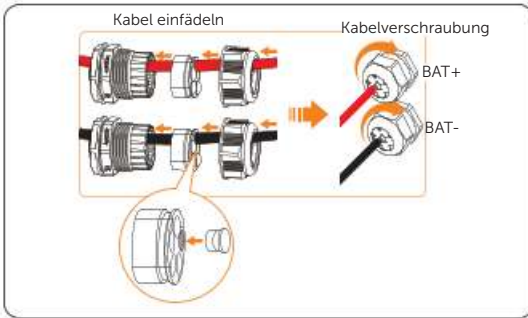
Abbildung 14-40 Stromkabel einfädeln
