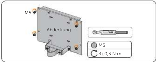
Abbildung 14-45 Abdeckung wieder anbringen
