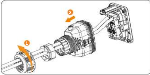
Abbildung 14-39 Netzwerkkabel entfernen
