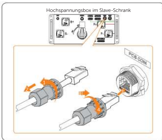
Abbildung 14-67 Kommunikationskabel einstecken
