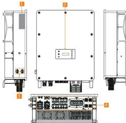
Abbildung 2-4 Teile-Beschreibung
