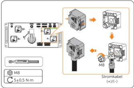
Abbildung 14-44 Stromkabel anschließen
