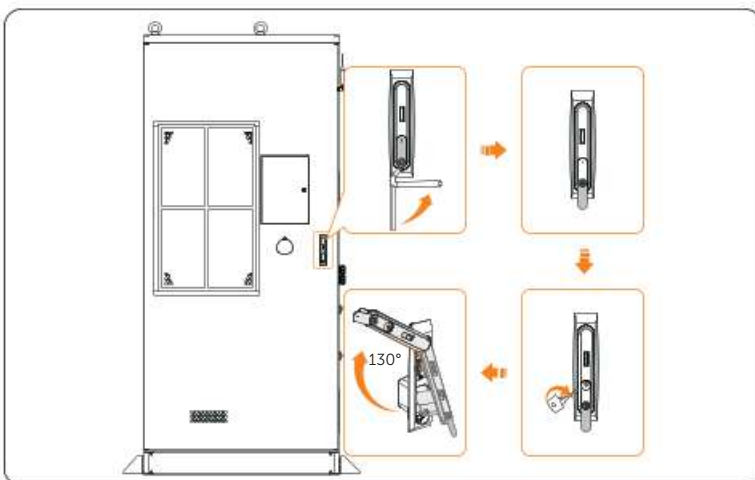
Abbildung 7-61 Vordertür öffnen
