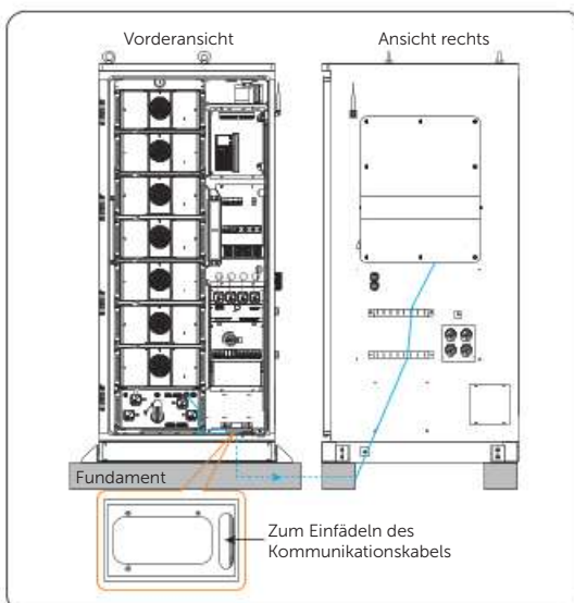
Abbildung 14-68 Kommunikationskabel einfädeln
