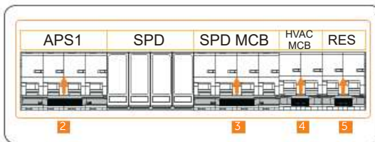
Abbildung 8-3 Schutzschalter hochklappen
