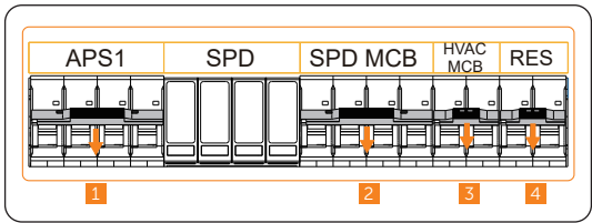
Abbildung 11-9 Schutzschalter herunterklappen
