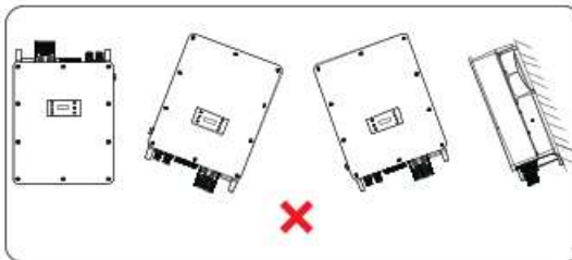
Abbildung 6-17 Falsche Installation
