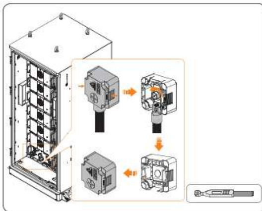
Abbildung 14-32 Stromkabel entfernen
