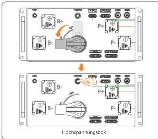
Abbildung 8-8 Hochspannungskasten starten
