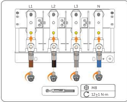
Abbildung 14-56 M8-Schrauben anziehen
