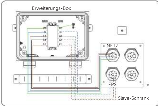
Abbildung 14-79 Schaltplan
