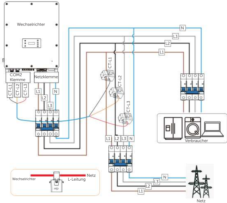
Abbildung 14-11 Systemverdrahtung mit CT
