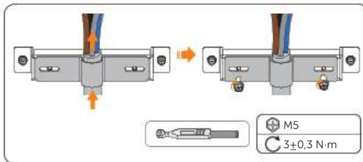
Abbildung 14-53 Netzdräht einfädeln
