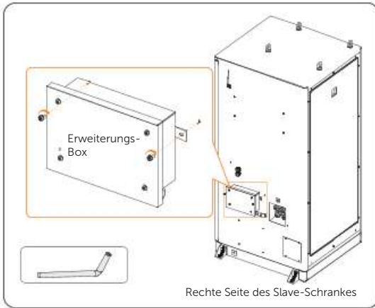
Abbildung 14-73 Erweiterungsbox installieren
