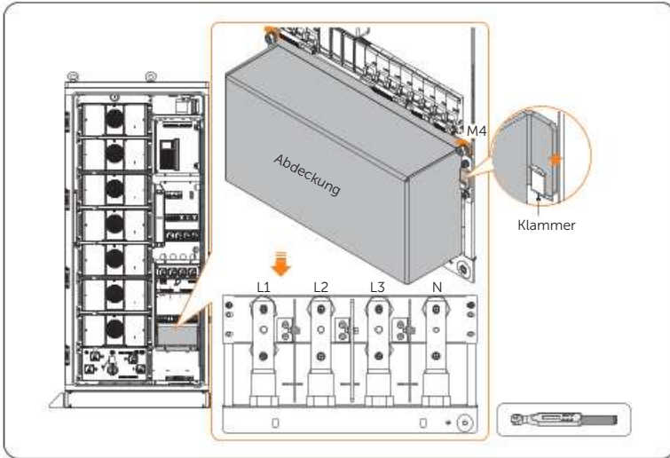
Abbildung 7-75 Abdeckung entfernen
