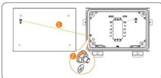
Abbildung 14-82 Erdungskabel wieder anschliessen
