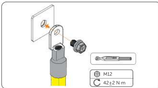
Abbildung 7-6 M12-Schrauben anziehen
