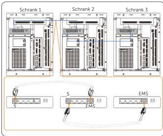
Abbildung 14-100 Ethernet-Kabel anschließen
