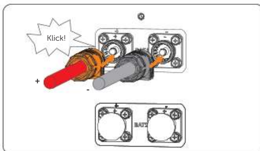
Abbildung 14-42 Montierte Batteriekabel anschließen
