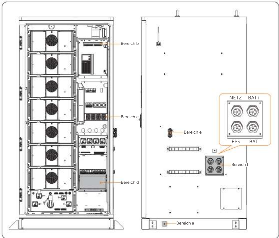
Abbildung 7-1 Verdrahtungsbereich
