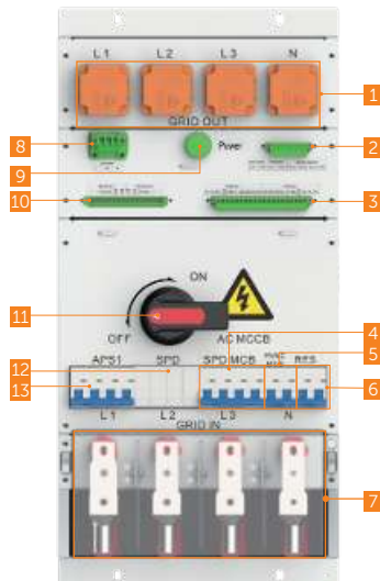
Abbildung 2-10 Frontplatte
