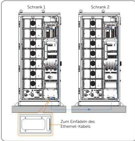
Abbildung 14-99 Ethernet-Kabel einfädeln
