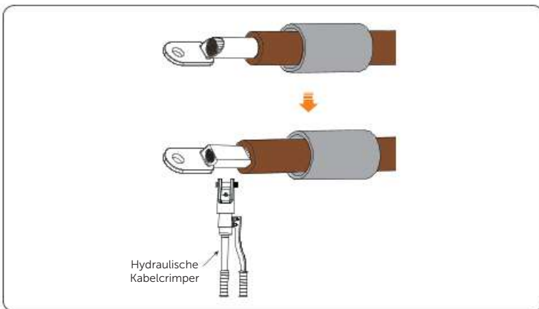
Abbildung 7-72 Crimpen
