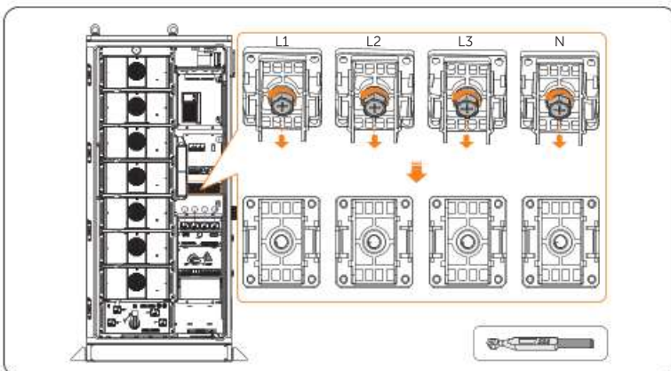
Abbildung 7-67 M8-Schrauben abschrauben
