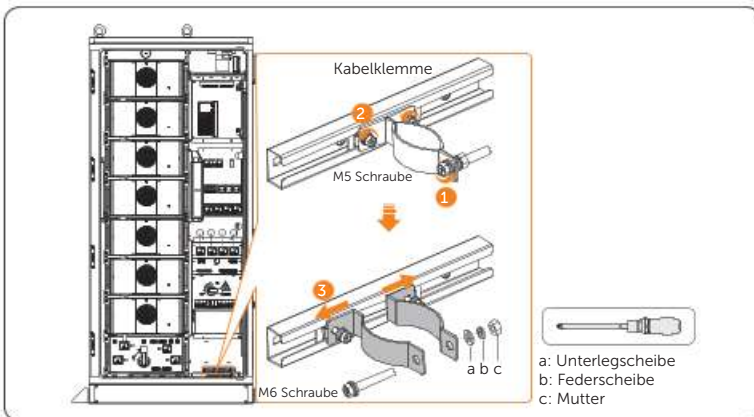
Abbildung 7-74 M6-Schrauben herausdrehen
