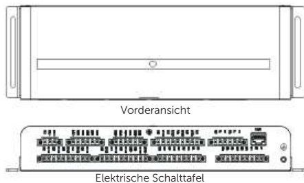
Abbildung 2-11 IO-Modul
