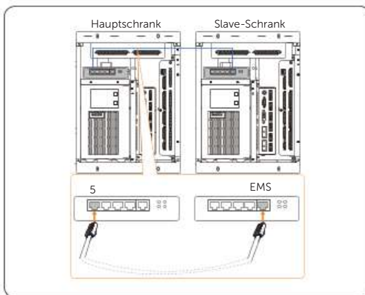
Abbildung 14-64 Ethernet-Kabel anschließen
