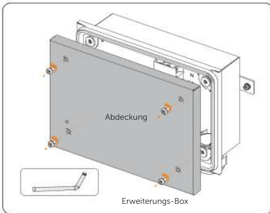
Abbildung 14-74 Gehäusedeckel entfernen
