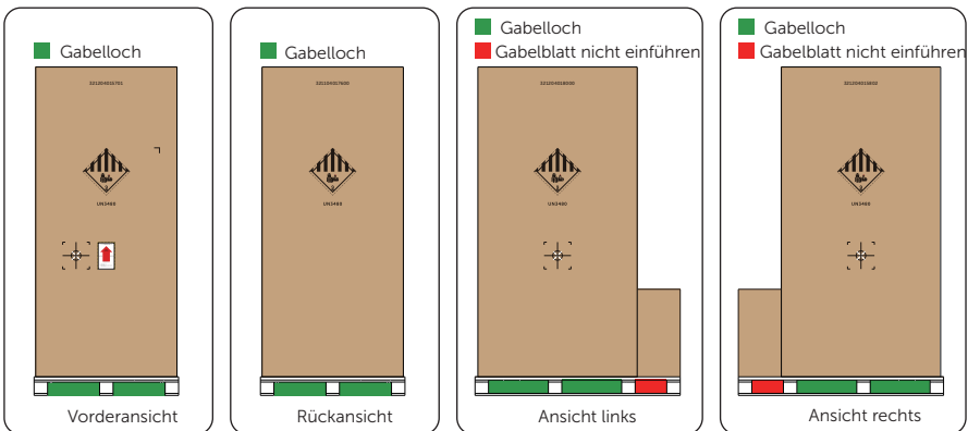
Abbildung 3-2 Karton-Gabel-Löcher
