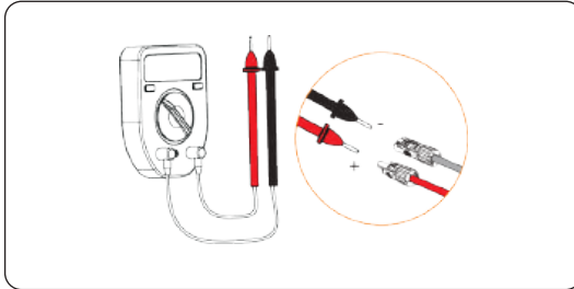
Abbildung 8-27 Spannung von PV-Steckverbindern messen
