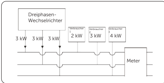
Abbildung 10-3 Phasen Unsymmetrie deaktiviert
