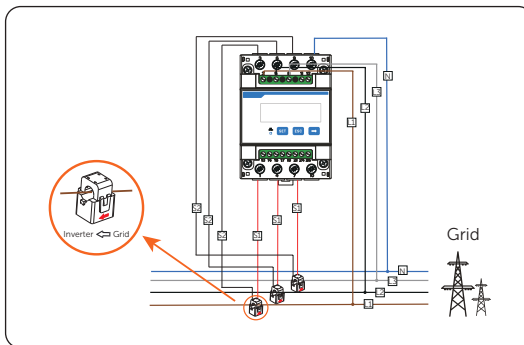
Abbildung 15-32 CT-angeschlossenes Meter an das Netz anschließen
