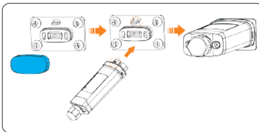
Abbildung 8-62 Den Dongle anschließen
