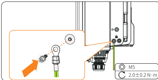
Abbildung 8-8 Das PE-Kabel sichern
