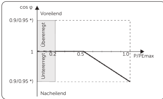
Abbildung 10-4 Kurve A
