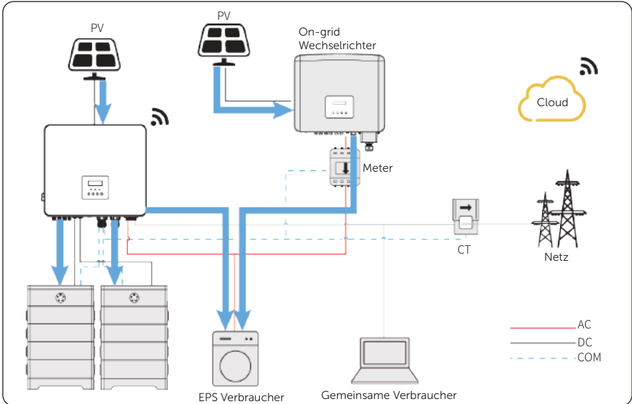
Abbildung 15-16 Stromfluss bei ausgeschaltetem Netz
