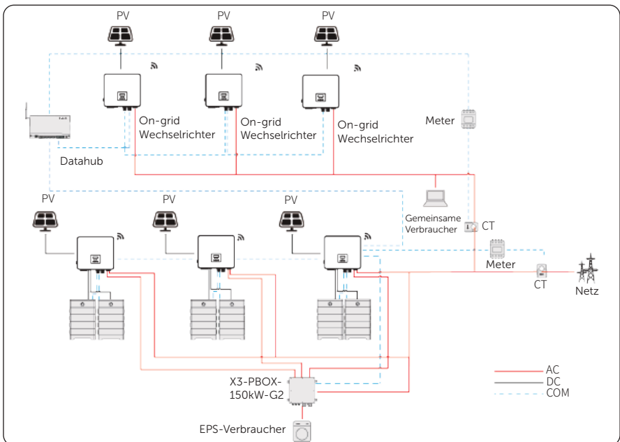
Abbildung 15-11 Schaltplan für DataHub
