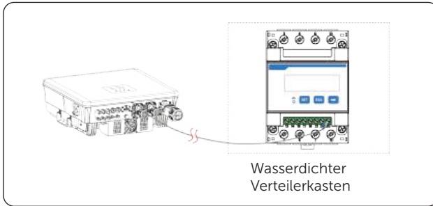
Abbildung 15-30 Wechselrichter an Solax Meter anschließen
