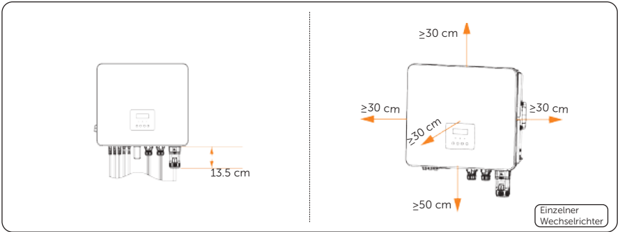
Abbildung 5-4 Abstandsanforderungen für einzelne Wechselrichter
