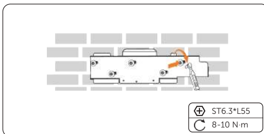
Abbildung 7-4 Die Halterung sichern
