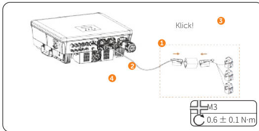
Abbildung 8-42 An Klemme COM 1 anschließen
