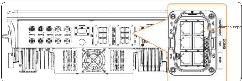
Abbildung 15-6 Anschlussklemme für Adapter Box
