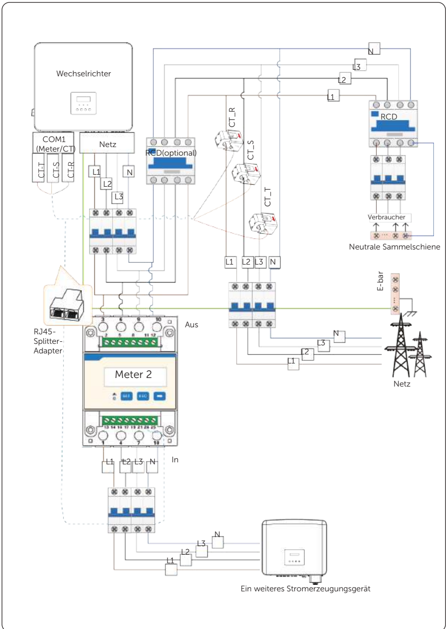
Abbildung 15-35 Anschlussplan von CT und direkt angeschlossenem Meter
