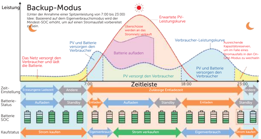
Abbildung 2-12 Backup-Modus
