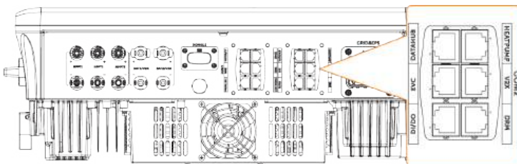
Abbildung 8-46 Gesamtaufbau der Klemme COM2
