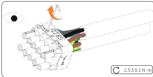
Abbildung 8-16 Das Netzkabel in den Gummikern einführen und festziehen
