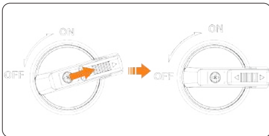
Abbildung 9-72 DC-Schalter entriegeln
