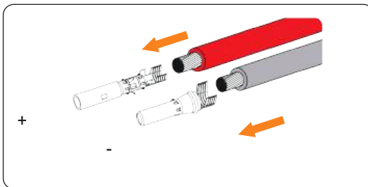
Abbildung 8-23 Den PV-Pin-Kontakt einsetzen
