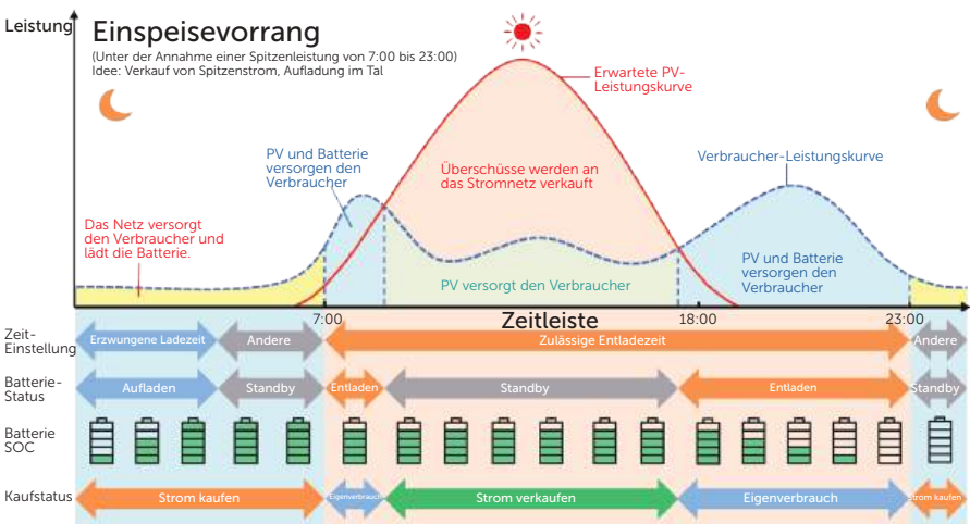
Abbildung 2-11 Einspeisevorrang
