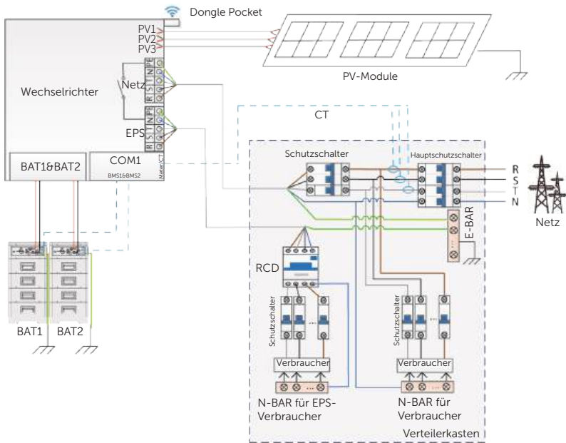
Abbildung 2-6 Partielles Home-Backup für Europa
