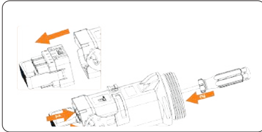
Abbildung 8-14 Den Gummikern herausdrücken
