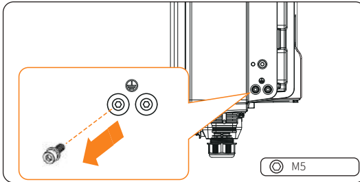
Abbildung 8-7 Die Schraube demontieren
