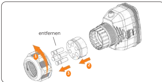
Abbildung 8-38 Das Gehäuse des Steckverbinders demontieren
