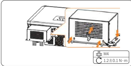
Abbildung 7-11 Kabelabschirmdeckel sichern
