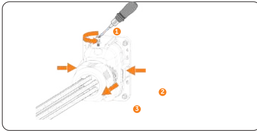
Abbildung 13-6 Den Kommunikations-Steckverbinder abtrennen
