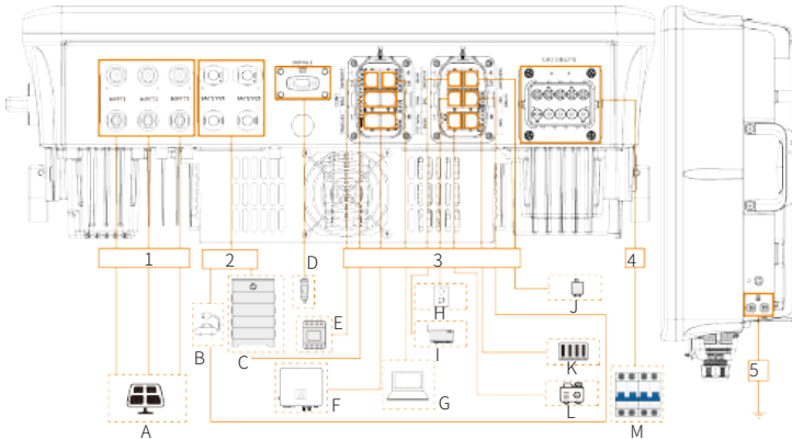
Abbildung 8-2 Kabelanschlüsse des Wechselrichters
