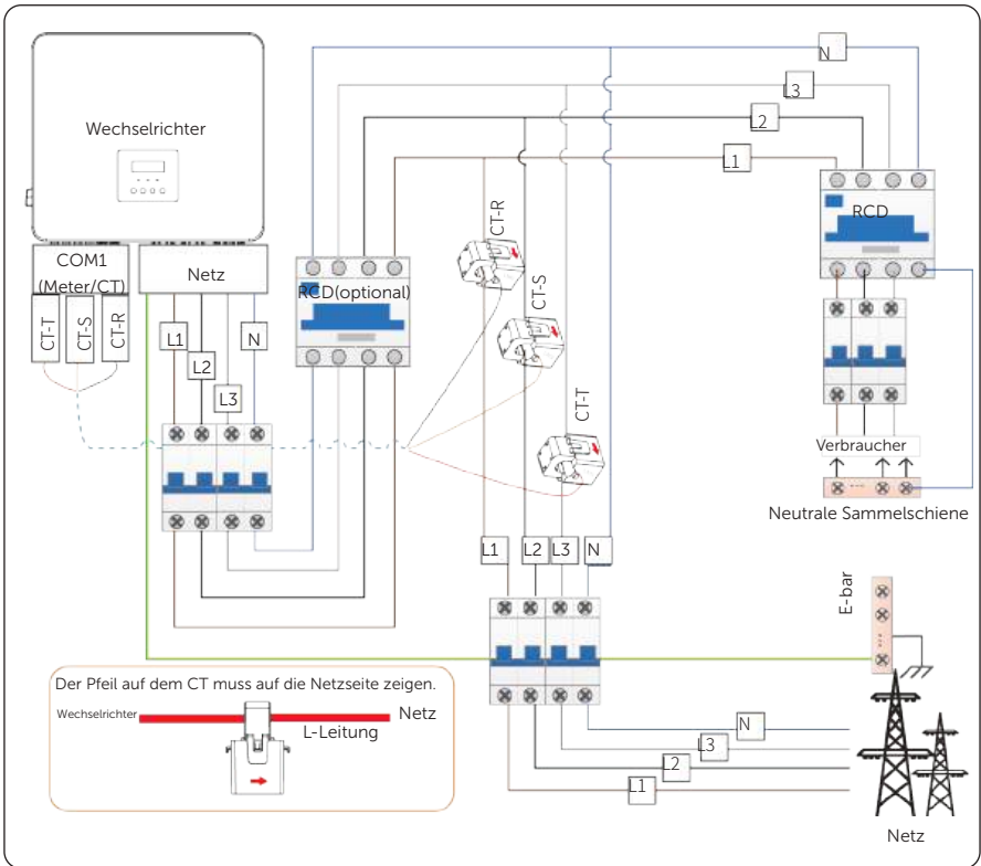
Abbildung 15-24 Systemverdrahtung mit CT
