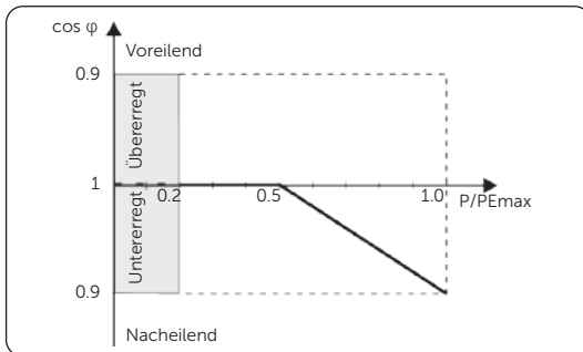
Abbildung 10-5 Kurve B
