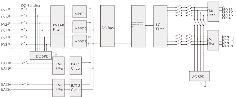
Abbildung 2-5 Stromlaufplan des Wechselrichters der Serie X3-HYB-G4 PRO
