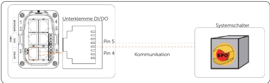
Abbildung 8-56 Anschlussplan für Systemschalter
