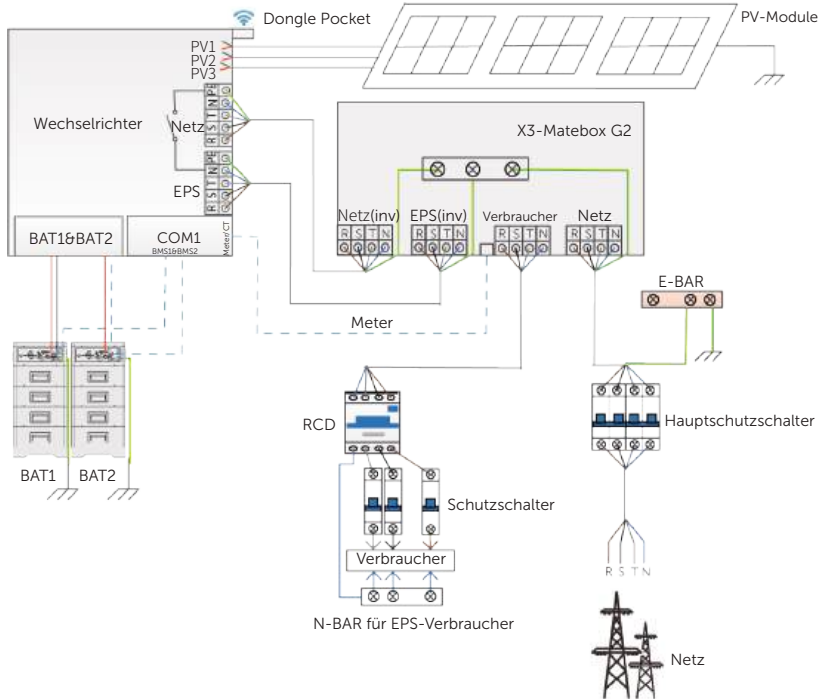
Abbildung 2-9 Vollständiges Home-Backup für Australien
