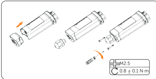
Abbildung 8-61 Den Dongle montieren
