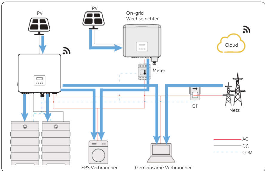
Abbildung 15-15 Stromfluss bei eingeschaltetem Netz und ausreichender PV
