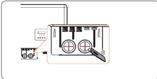
Abbildung 7-9 Den Drahtschutzring durchschneiden
