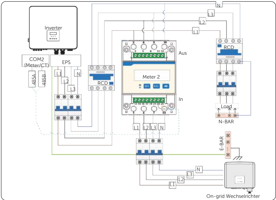
Abbildung 15-17 Anschlussplan von Meter an EPS-Klemme
