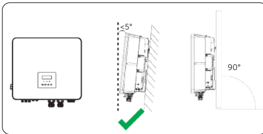
Abbildung 7-1 Korrekte Installation
