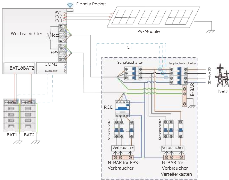
Abbildung 2-8 Partielles Home-Backup für Australien
