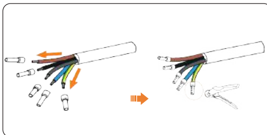
Abbildung 8-10 Kern und Aderendhülse zusammencrimpen
