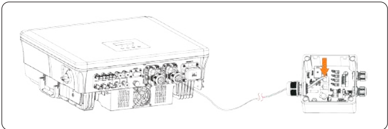
Abbildung 15-7 An Adapter Box G2 anschließen
