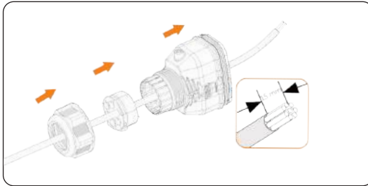
Abbildung 8-40 Das Kabel ohne RJ45-Klemme einfädeln und abisolieren
