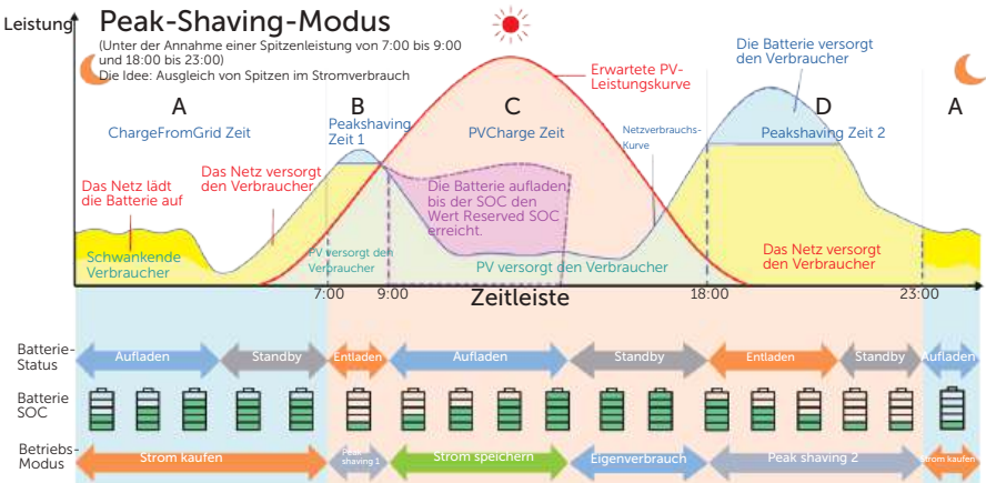
Abbildung 2-13 Peak-Shaving-Modus
