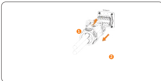
Abbildung 13-5 Die Verriegelung nach oben ziehen und den Steckverbinder herausziehen
