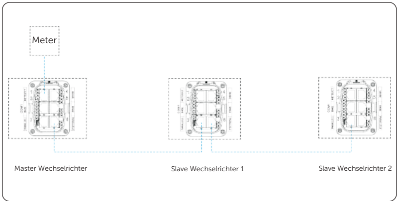
Abbildung 15-23 Kommunikationsverdrahtung ohne X3-PBOX-150kW-G2
