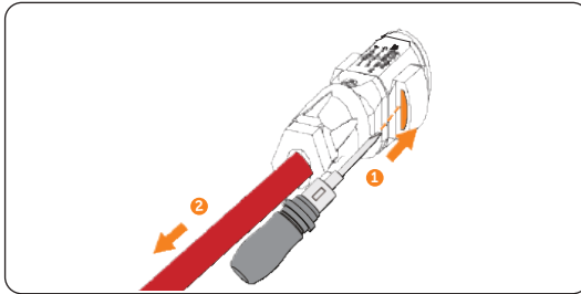
Abbildung 13-3 Batterie-Steckverbinder abtrennen
