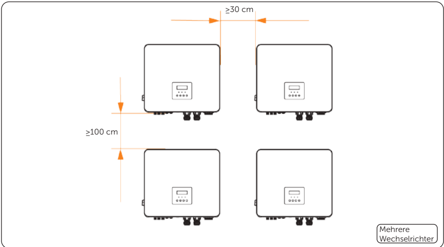
Abbildung 5-5 Abstandsanforderungen für mehrere Wechselrichter
