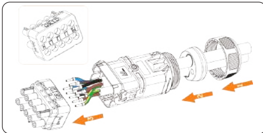
Abbildung 8-15 Leiter einfädeln und festziehen
