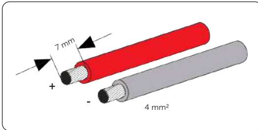
Abbildung 8-22 PV-Kabel abisolieren
