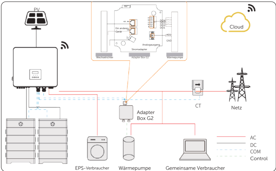
Abbildung 15-4 Schaltplan für Adapter Box G2
