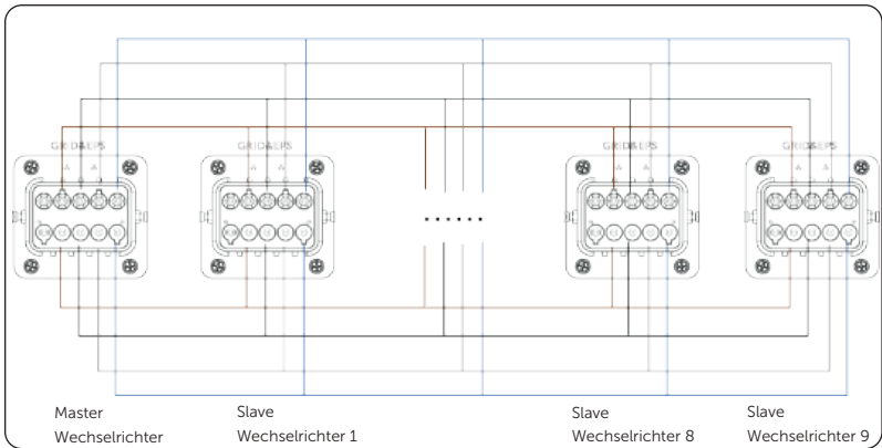
Abbildung 15-20 Stromkabel-Verdrahtung mit X3-PBOX-150kW-G2
