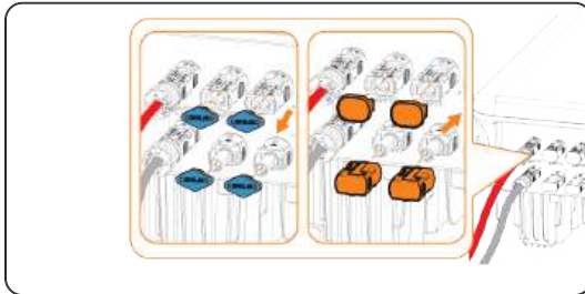
Abbildung 8-29 Ungenutzte Klemmen mit Schnallen verschließen
