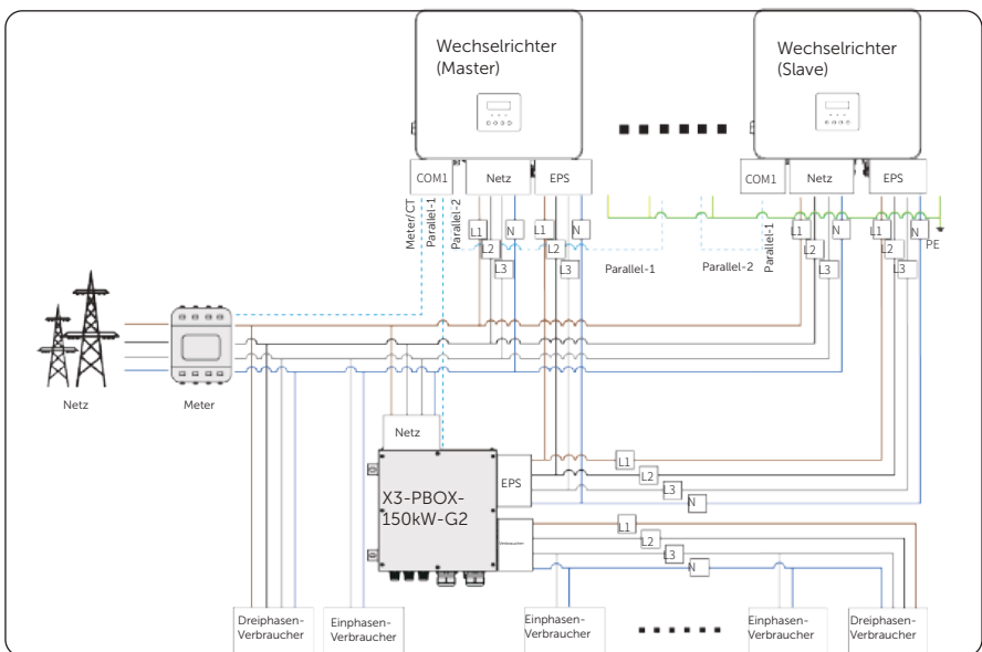
Abbildung 15-18 Mit X3-PBOX-150kW-G2 System-Schaltplan
