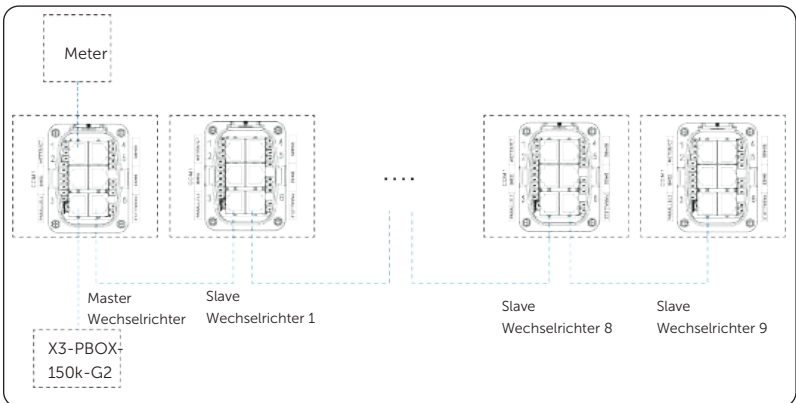
Abbildung 15-22 Kommunikationsverdrahtung mit X3-PBOX-150kW-G2
