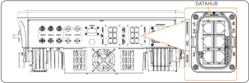
Abbildung 15-12 Anschlussklemme für DataHub
