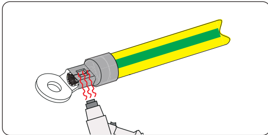
Abbildung 8-6 Den Schlauch schrumpfen
