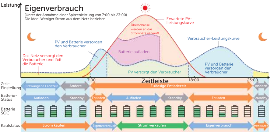
Abbildung 2-10 Eigenverbrauch-Modus
