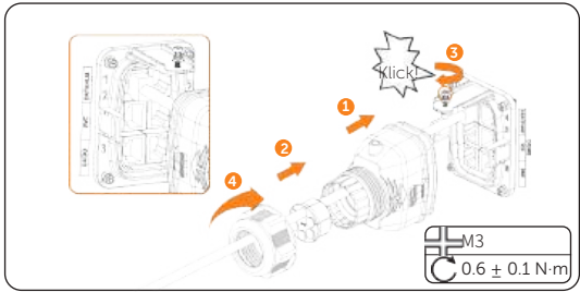
Abbildung 8-52 An die Klemme COM 2 anschließen
