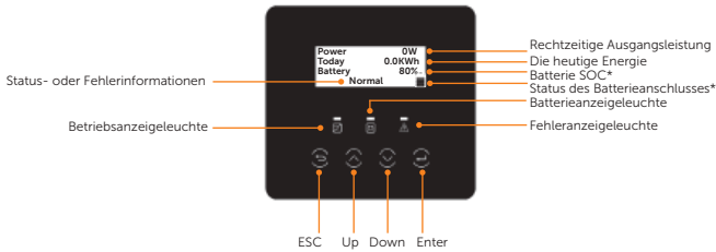
Abbildung 10-1 Bedienfeld
