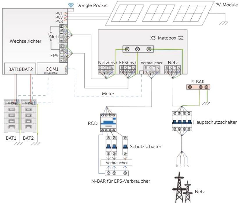
Abbildung 2-7 Vollständiges Home-Backup für Europa
