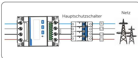
Abbildung 15-28 Direkt angeschlossener Meter an das Netz anschließen
