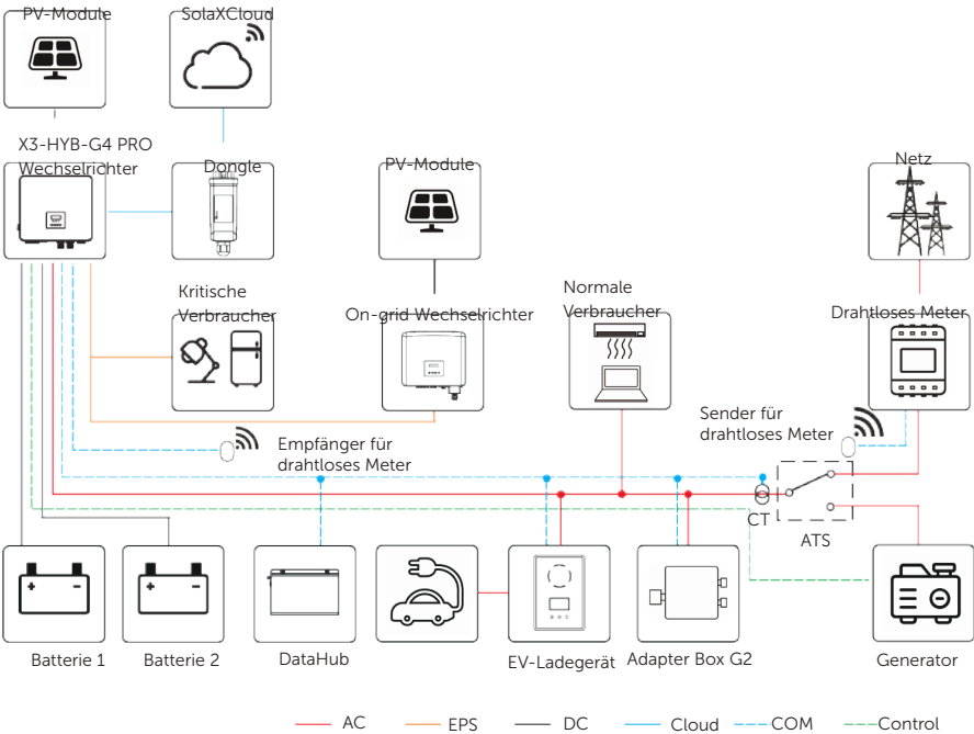
Abbildung 3-1 Systemdiagramm
