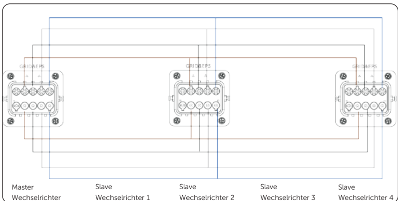
Abbildung 15-21 Stromkabel-Verdrahtung ohne X3-PBOX-150kW-G2
