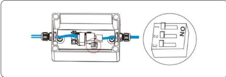
Abbildung 15-5 DIP-Schalter in OFF -Position
