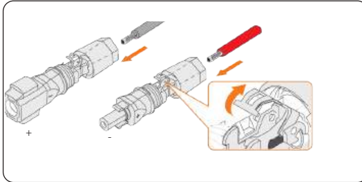
Abbildung 8-31 Das Kabel in den Batterie-Steckverbinder einföhren
