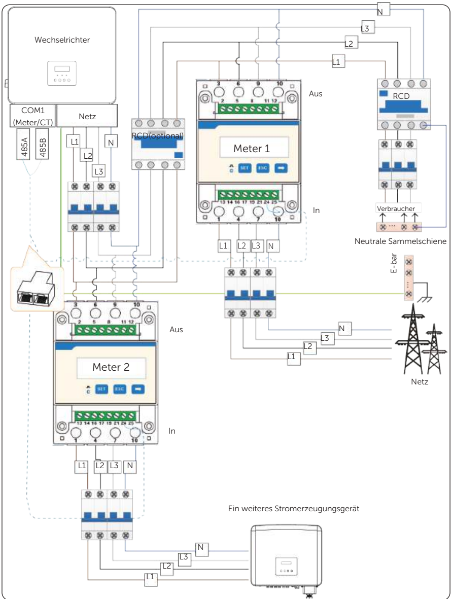
Abbildung 15-36 Anschlussplan von zwei direkt angeschlossenen Metern
