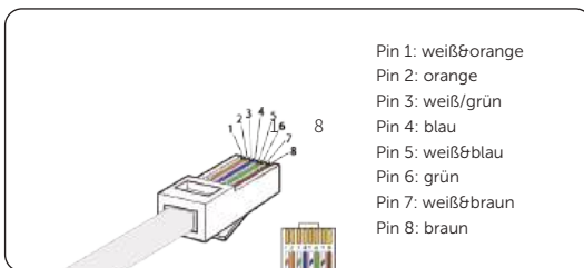
Abbildung 8-51 Die Signalkabel einföhren und das Kabel crimpen
