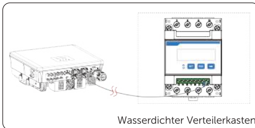
Abbildung 8-44 An SolaX Meter anschließen
