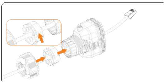
Abbildung 8-39 Das Kabel mit der RJ45-Klemme einfädeln
