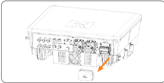
Abbildung 8-19 Die Kappe entfernen
