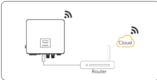
Abbildung 8-60 Anschlussplan für den LAN-Modus
