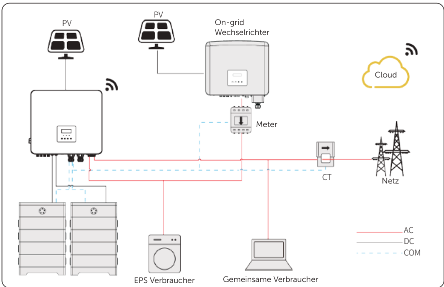
Abbildung 15-14 Schaltplan für Mikro-Netz
