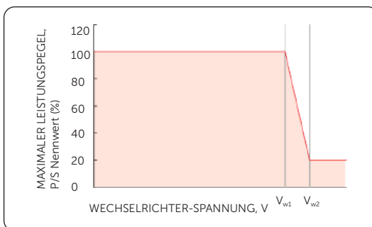
Abbildung 10-7 Kurve für P(u)
