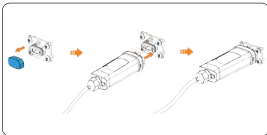
Abbildung 8-65 Den Dongle anschließen
