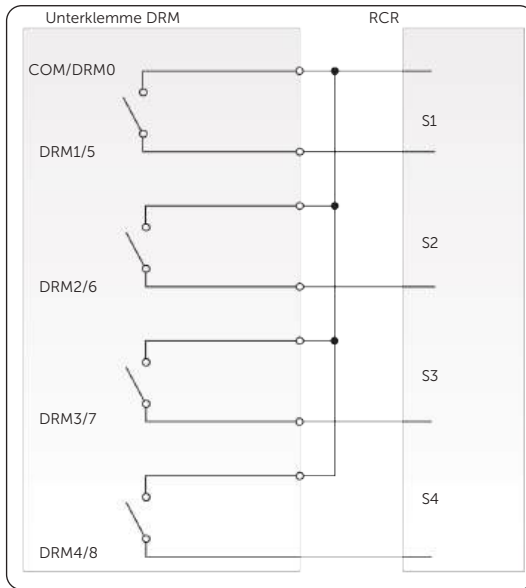
Abbildung 8-58 RCR-Anschlussplan
