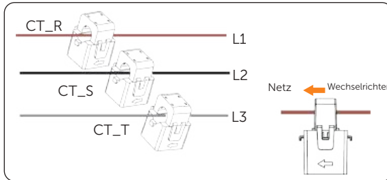
Abbildung 15-25 CTs an Netzkabel klemmen
