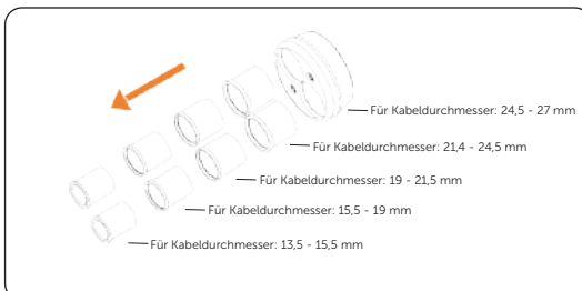
Abbildung 8-13 Verschlussstopfen herausnehmen
