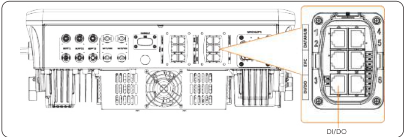
Abbildung 15-3 Anschlussklemme für Generator
