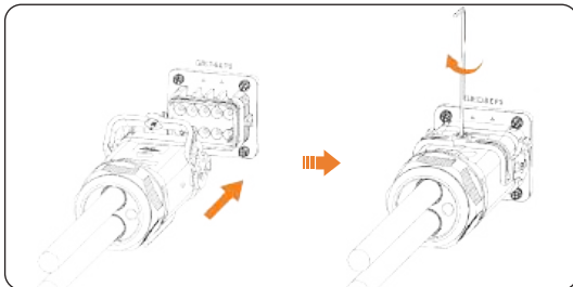
Abbildung 8-21 AC-Steckverbinder in die Klemme einstecken und verriegeln
