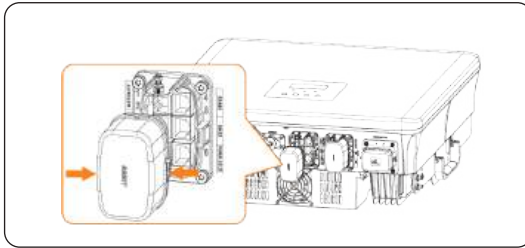
Abbildung 8-37 Die staubdichte Abdeckung entfernen
