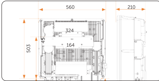
Abbildung 7-3 Abmessungen (Einheit: mm)
