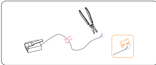
Abbildung 15-33 Kommunikationskabel für Meter abisolieren
