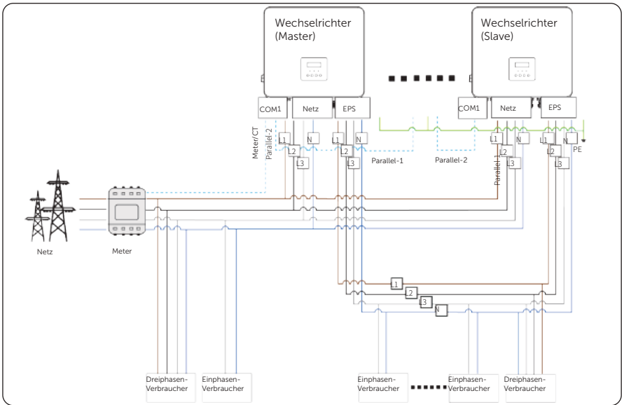
Abbildung 15-19 Ohne X3-PBOX-150kW-G2 System-Schaltplan
