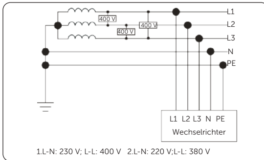
Abbildung 2-3 Unterstütztes Stromnetz: TN-S
