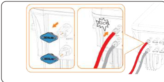
Abbildung 8-28 Das PV-Kabel anschließen
