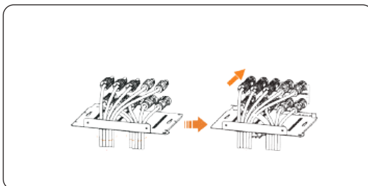
Abbildung 7-10 Kabel sortieren und einfädeln
