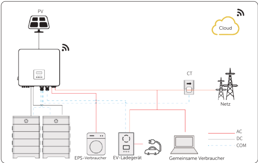
Abbildung 15-8 Schaltplan für EV-Ladegerät
