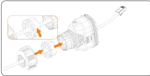
Abbildung 8-49 Das Kabel mit der RJ45-Klemme einfädeln
