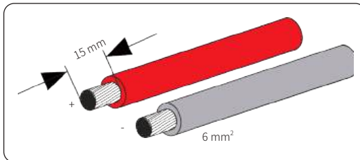
Abbildung 8-30 Das Batteriekaabel abisolieren
