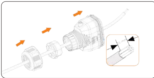
Abbildung 8-50 Das Kabel ohne RJ45-Klemme einfädeln und abisolieren
