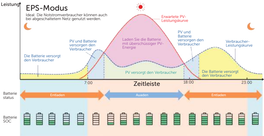
Abbildung 2-14 EPS-Modus
