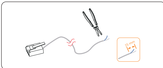
Abbildung 15-29 Kommunikationskabel für Meter abisolieren
