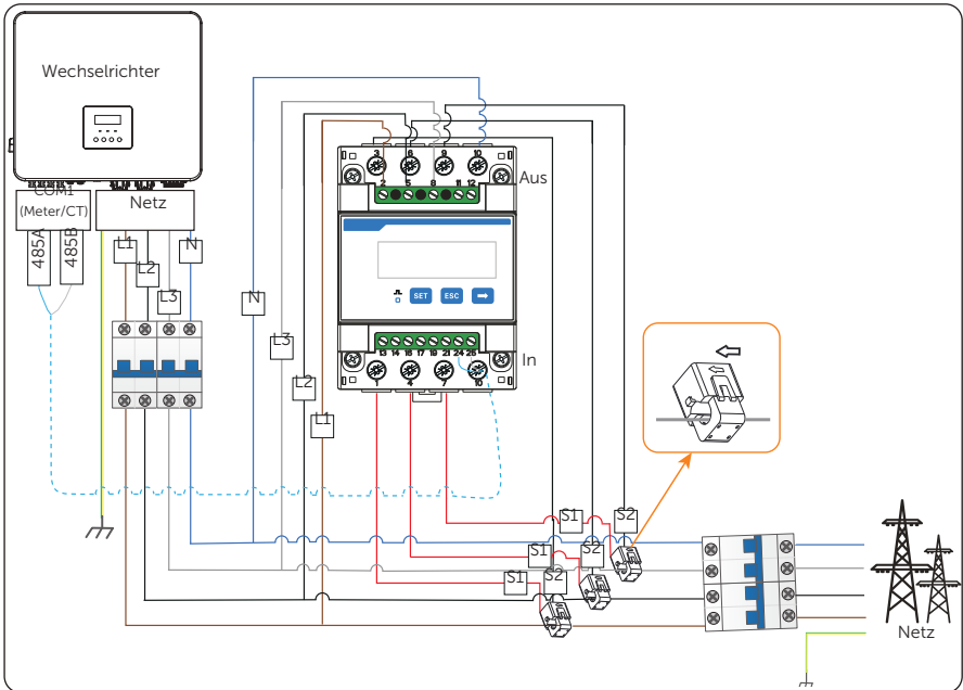
Abbildung 15-31 Systemverdrahtung mit SolaX CT-angeschlossenem Meter
