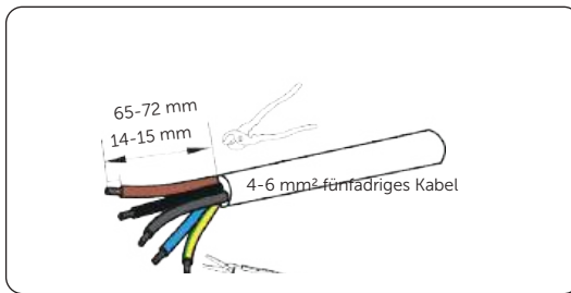
Abbildung 8-9 Netz- und EPS-Kabel abisolieren
