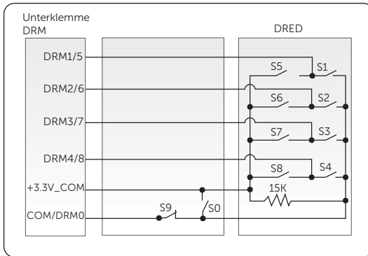
Abbildung 8-57 DRED-Anschlussplan
