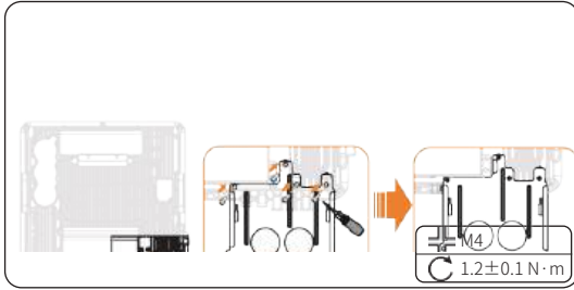
Abbildung 7-1 Die Halterung montieren
