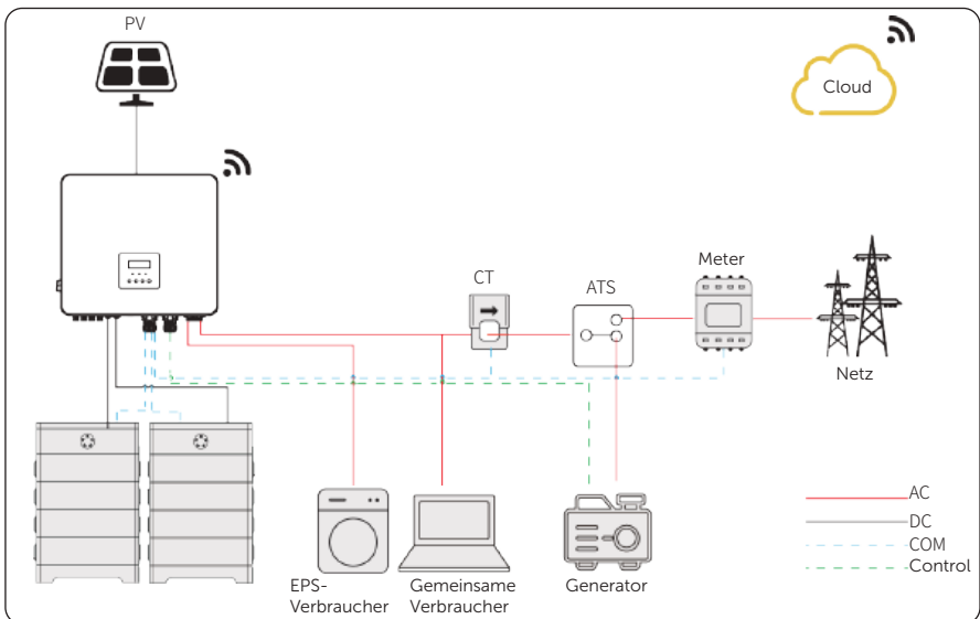
Abbildung 15-2 Schaltplan für Potentialfreier Kontakt
