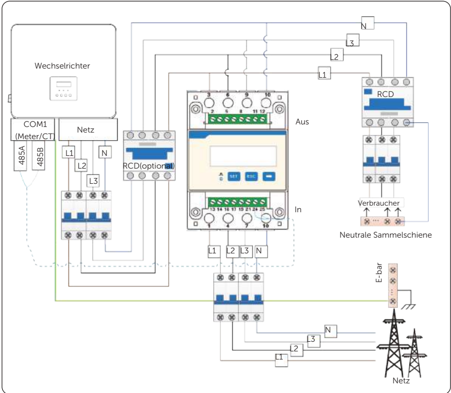
Abbildung 15-27 Systemverdrahtung mit direkt angeschlossenen Meter
