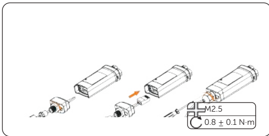
Abbildung 8-64 Den Dongle montieren
