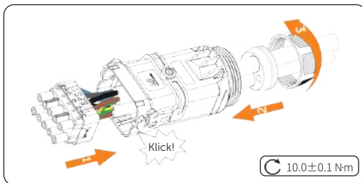
Abbildung 8-18 AC-Steckverbinder montieren
