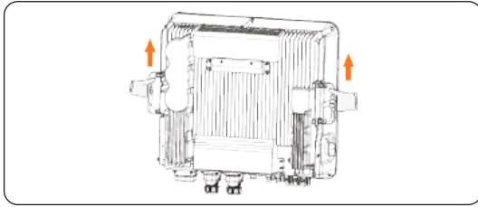
Abbildung 7-5 Die Griffe herausziehen und das Gerät anheben
