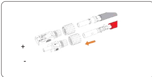
Abbildung 8-25 Das PV-Kabel einfädeln
