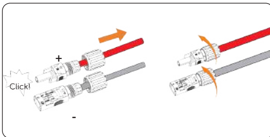
Abbildung 8-26 Das PV-Kabel sichern
