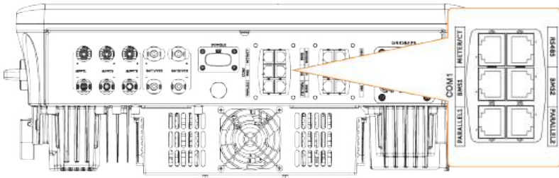
Abbildung 8-36 Gesamtaufbau der Klemme COM 1
