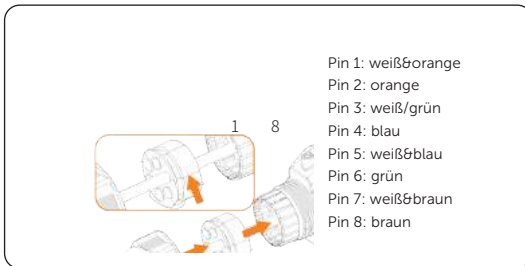
Abbildung 8-41 Die Signalkabel einföhren und das Kabel crimpen
