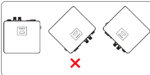
Abbildung 7-2 Falsche Installation
