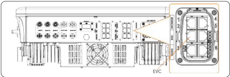
Abbildung 15-9 Anschlussklemme für EV-Ladegerät
