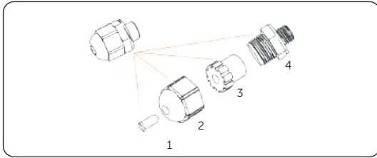
Abbildung 8-63 Den wasserdichten Steckverbinder demontieren
