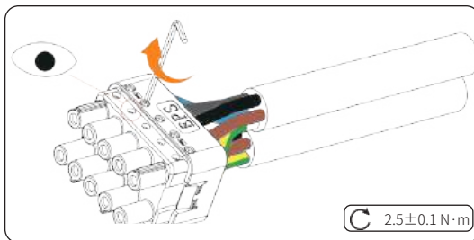
Abbildung 8-17 Das EPS-Kabel in den Gummikern einführen und festziehen
