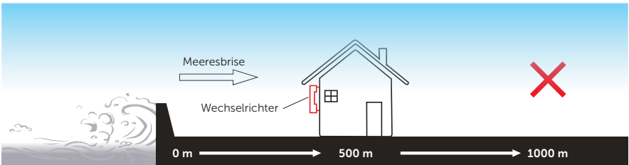
Abbildung 5-2 Falsche Einbaulage
