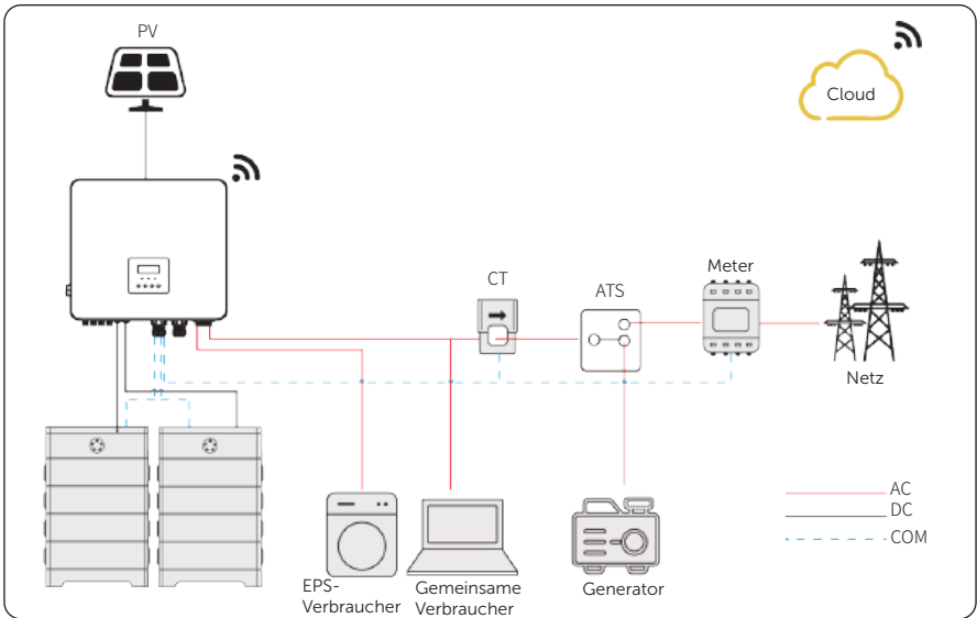
Abbildung 15-1 Schaltplan für ATS-Steuerung
