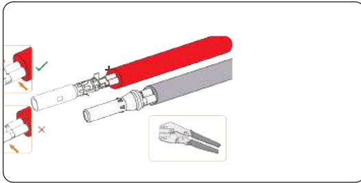
Abbildung 8-24 Die Klemme crimpen
