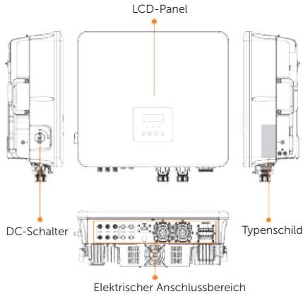
Abbildung 2-1 Erscheinungsbild
