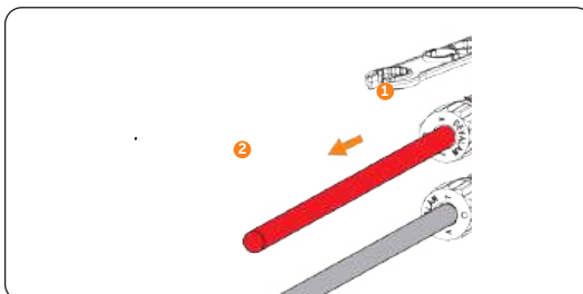
Abbildung 13-2 PV-Steckverbinder abtrennen
