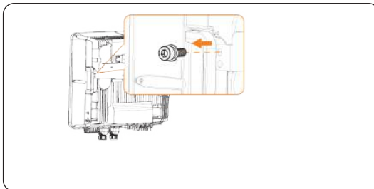
Abbildung 13-7 Die M5-Schraube entfernen
