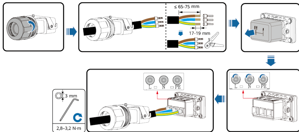
Abbildung 5-4 Anschließen des AC-Stromkabels
