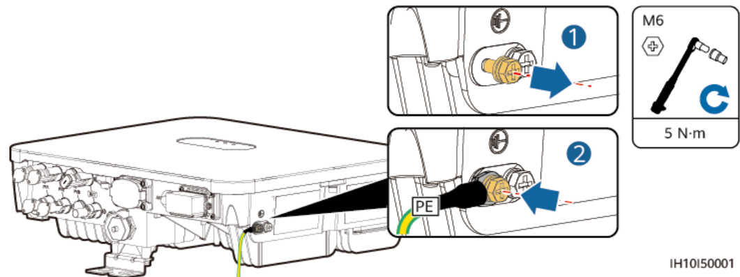
Abbildung 5-3 Anschließen des PE-Kabels
