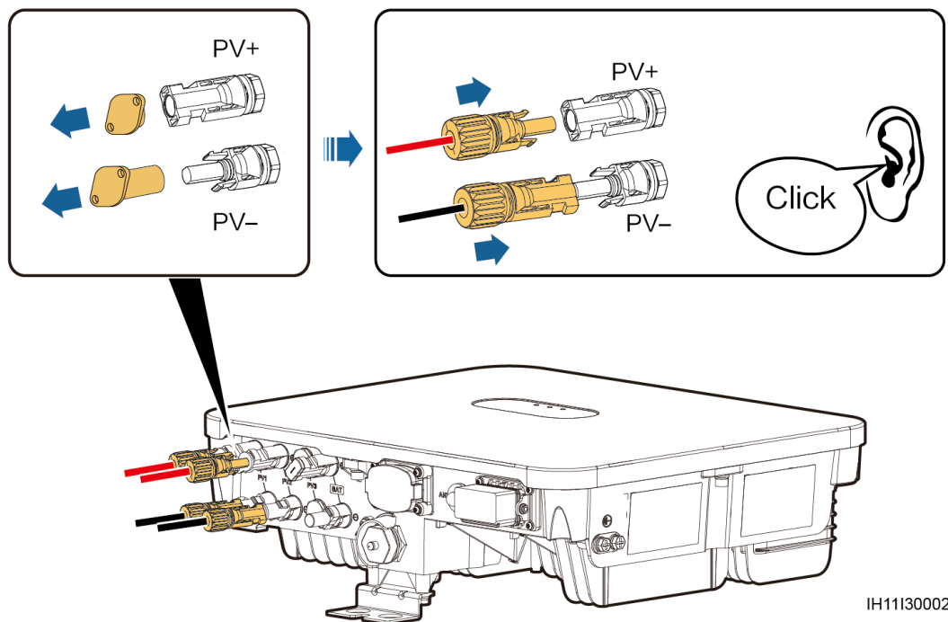
Abbildung 5-10 Anschließen der DC-Eingangsstromkabel
