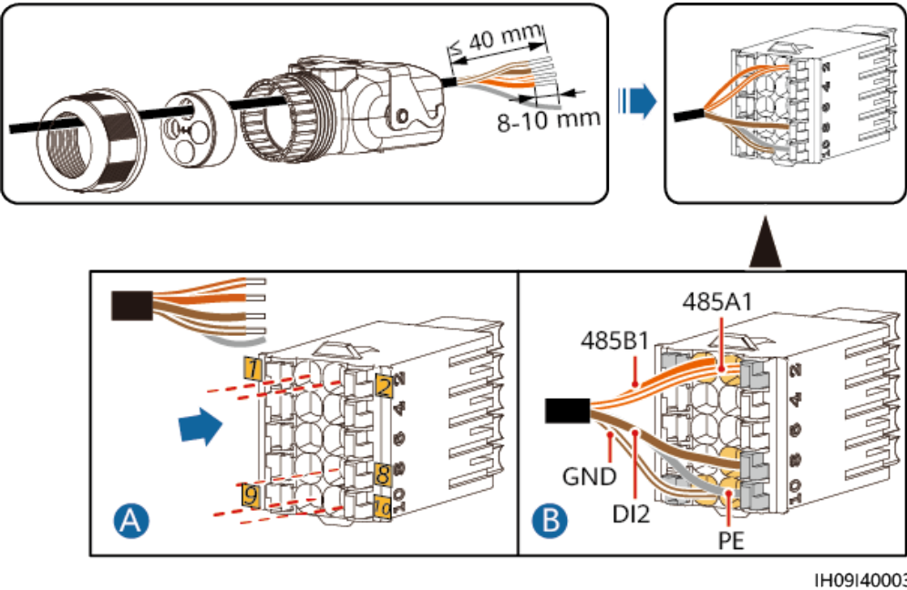
Abbildung 5-25 Anschließen der Kabel (Verbinden mit SmartGuard)
