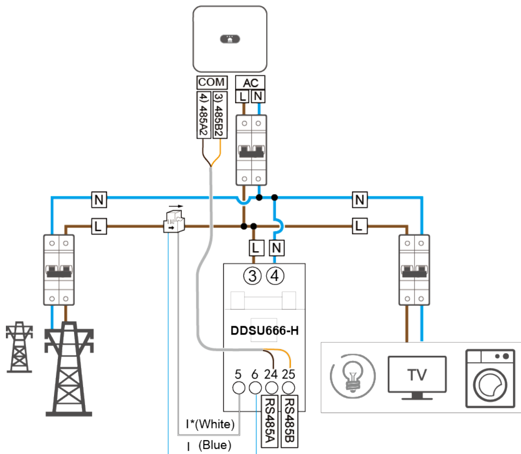
Abbildung 5-28 Anschluss von Kabeln an den Stromzähler DDSU666-H
