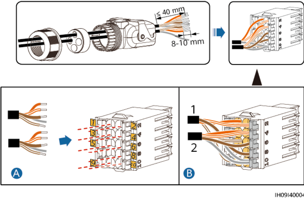
Abbildung 5-26 Installieren von Kabeln
