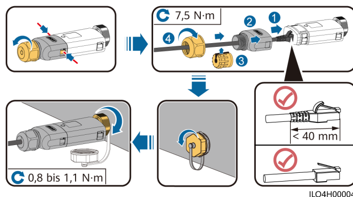
Abbildung 5-46 Installieren von WLAN-FE-Smart Dongle (FE-Kommunikation)
