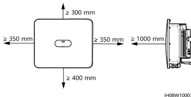
Abbildung 4-2 Abstände
