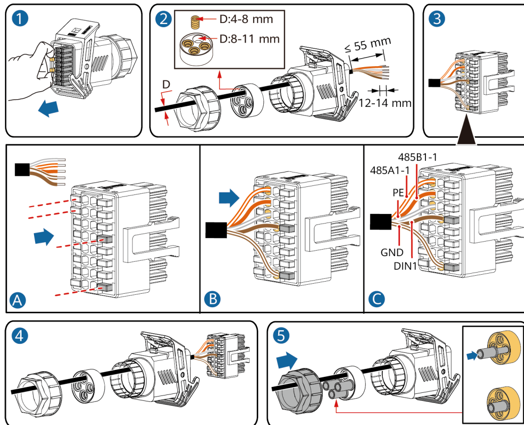
Abbildung 5-34 Kabelmontage
