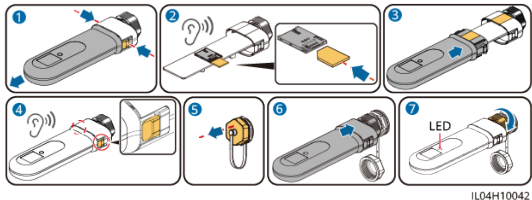
Abbildung 5-48 Installieren von 4G Smart Dongle (SDongleB-06)
