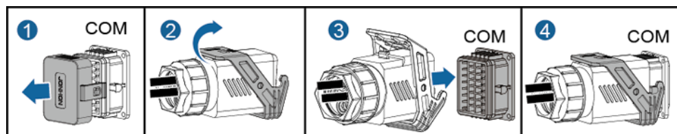
Abbildung 5-33 Sichern des Signalkabelsteckverbinders
