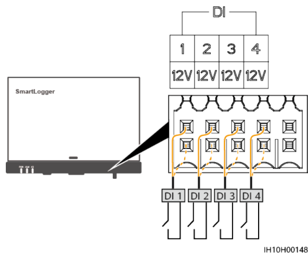
Abbildung 5-39 Kabelverbindungen (SmartLogger-Vernetzung)
