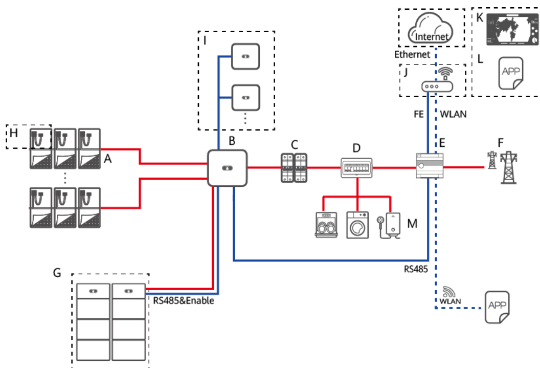
Abbildung 2-3 SmartAssistant-Vernetzung (die Komponenten in den gestrichelten Kästen sind optional)
