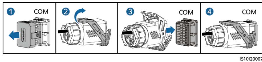
Abbildung 5-37 Sichern des Signalkabelanschlusses
