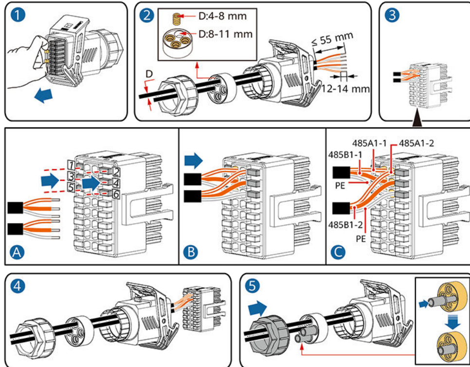
Abbildung 5-21 Kabelmontage
