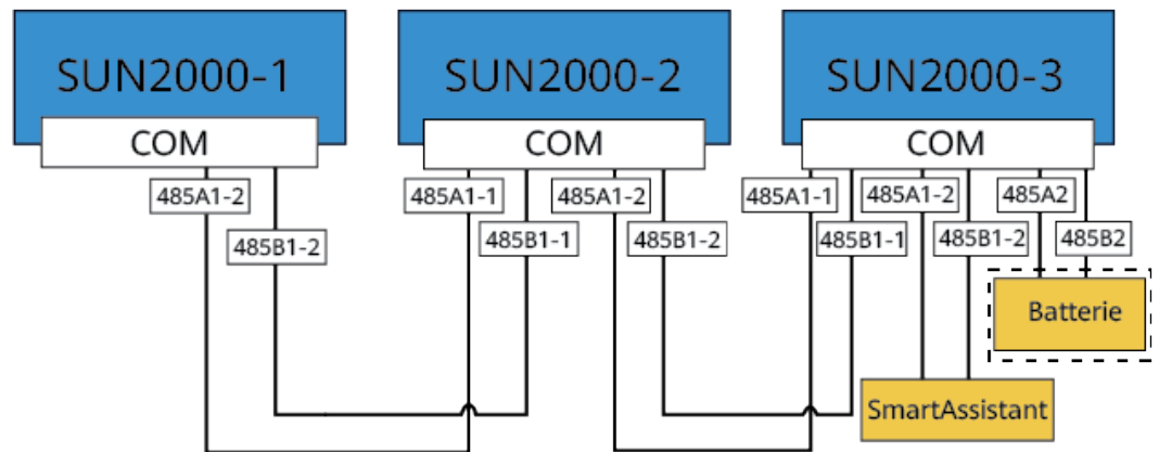
Abbildung 5-19 SmartAssistant-Vernetzung (die Komponente im gestrichelten Kasten ist optional)
