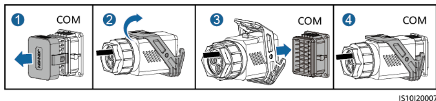
Abbildung 5-31 Sichern des Signalkabelsteckverbinders
