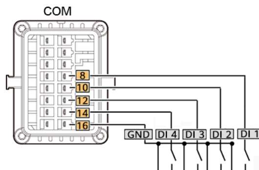
Abbildung 5-38 Kabelverbindungen (Smart Dongle-, SmartAssistant- und SmartGuard-Vernetzung)
