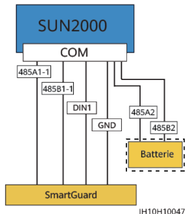
Abbildung 5-20 SmartGuard-Vernetzung (die Komponente im gestrichelten Kasten ist optional)
