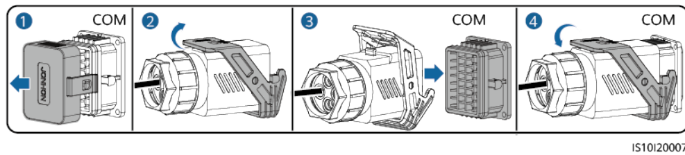
Abbildung 5-41 Sichern des Signalkabelsteckers
