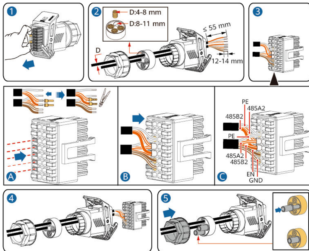
Abbildung 5-28 Installieren von Kabeln
