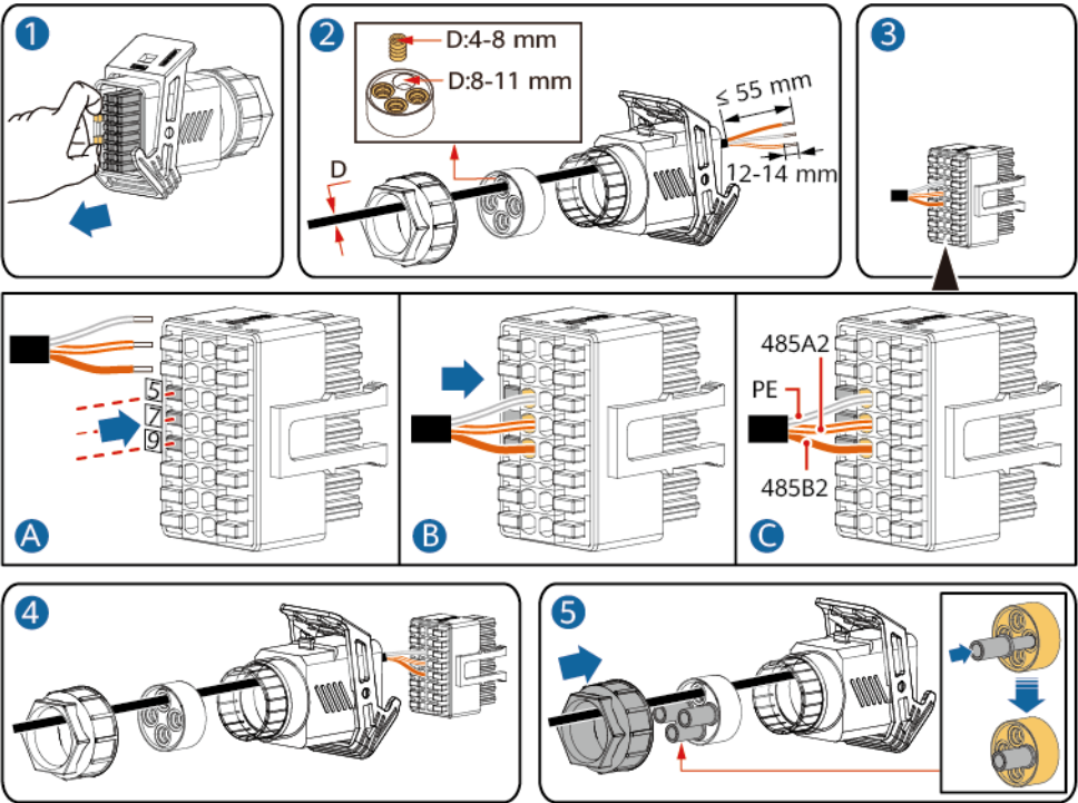
Abbildung 5-26 Kabelmontage
