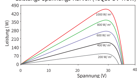
Leistungs-Spannungs-Kurven (48QL6-DV 475W)
