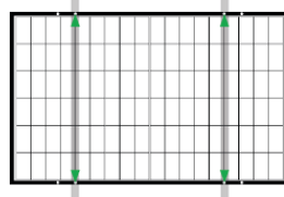
Abb. 8 Nutzung der vier Bohrungen, Schienen orthogonal zur langen Rahmenseite
