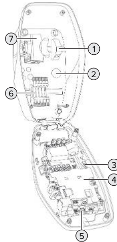
Kuva 3: Sisänäkymä (esimerkki)
