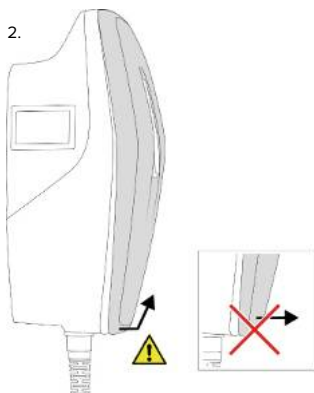
Fig. 5: Desmontar la cubierta frontal - 2
