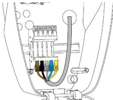
Fig. 10: Tilslutning strømforsyning (eksempel)
