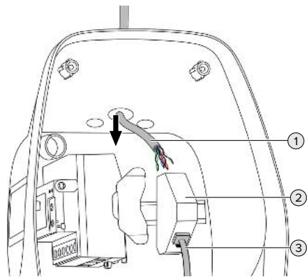
15. Ábra: Adatkábel csatlakoztatása (példa)
