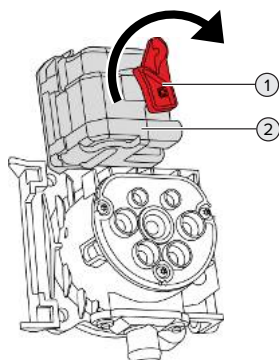
Fig. 25 : Déverrouillage manuel de la fiche de charge
