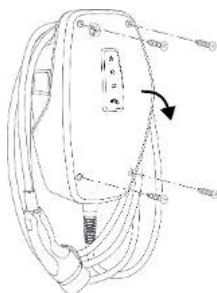
Fig. 6: Åbne produktet (eksempel)
