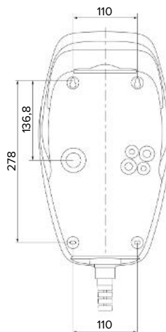
Fig. 7: Dimensioni dei fori [mm]
