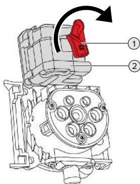
Fig. 25: Sblocco manuale della spina di ricarica
