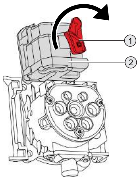
Abb. 25: Ladestecker manuell entriegeln
