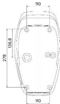
Kuva 8: Porausmitat [mm]
