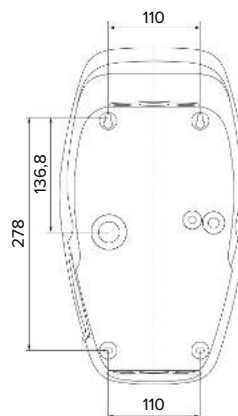
Fig. 8: Dimensioni dei fori [mm]
