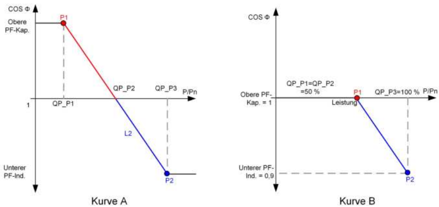
Abbildung 7-19 Blindleistungsregulierungskurve im Q(P)-Modus
