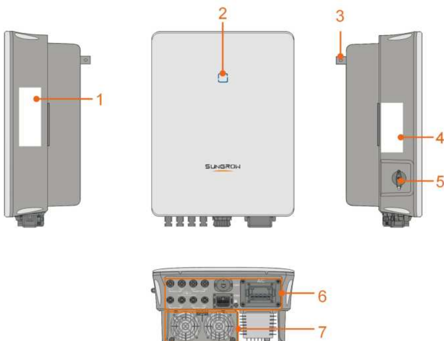
Abbildung 2-2 Wechselrichter Erscheinungsbild
