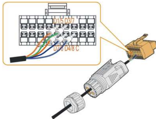
Abbildung 5-10 DI-Verbindung
