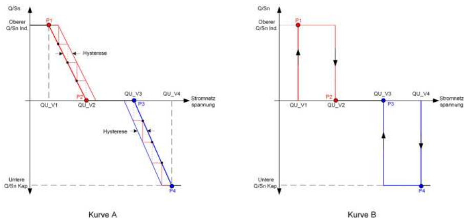
Abbildung 7-20 Blindleistungsregelungskurve in Q(U)-Kurve
