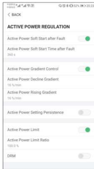
Abbildung 7-17 Wirkleistungsregelung
