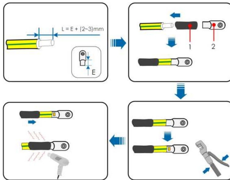
(1) Schrumpfschlauch
