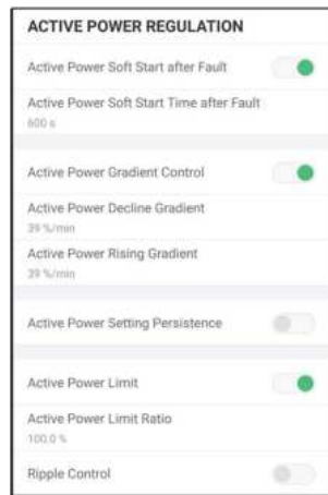
Abbildung 8-18 Regelung Wirkleistung
